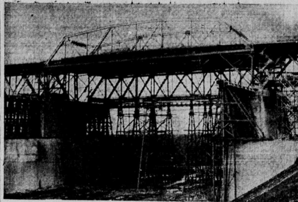
NOUVELLE TRAVEE EN PLACE — Le Pont Jacques-Cartier a, depuis dimanche matin, un nouveau profil dans son tronçon près de la rive sud. Voici en effet la nouvelle travée qui a été posée hier, pour permettre une hauteur libre suffisante pour le canal du Saint-Laurent.
