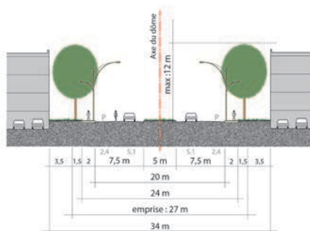
Collectrice centrale, 3 étages (au nord du parc)
