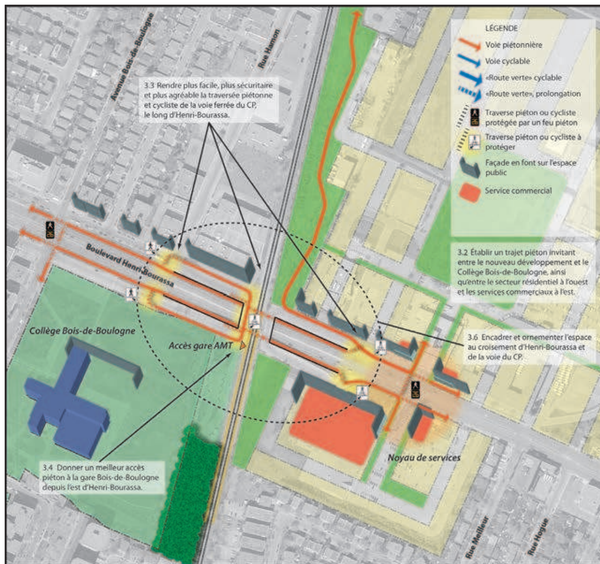
Plan 7.12 : Actions pour le passage de la voie du CP : Option sous le viaduc, piétons
