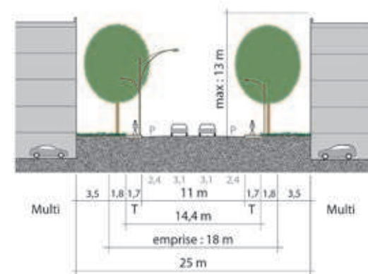
Collectrice, ouest du parc, 4 étages (rue Dazé)
