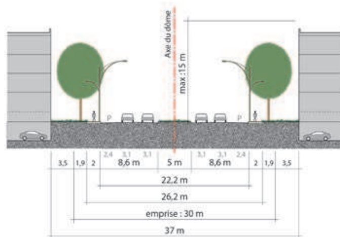
Collectrice centrale, 4 étages (au sud du parc)
