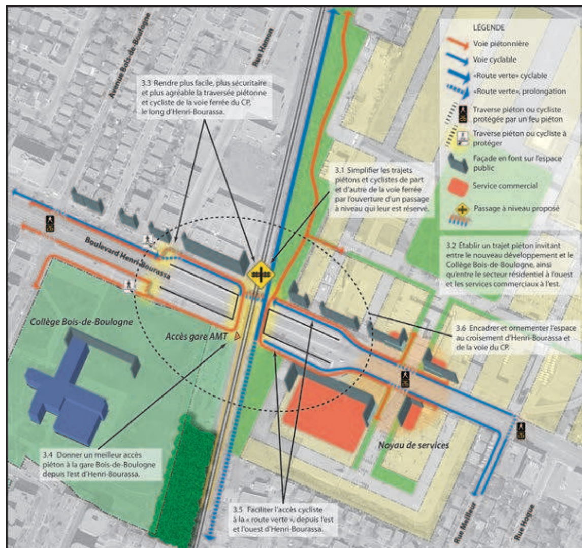
Plan 7.11 : Actions pour le passage de la voie du CP : Option passage à niveau
