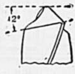
B Angle de dégagement des lèvres
