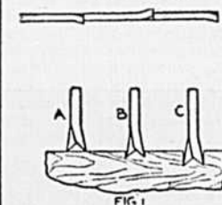
Comment aiguïser les scies de travers ("cross-cut")
