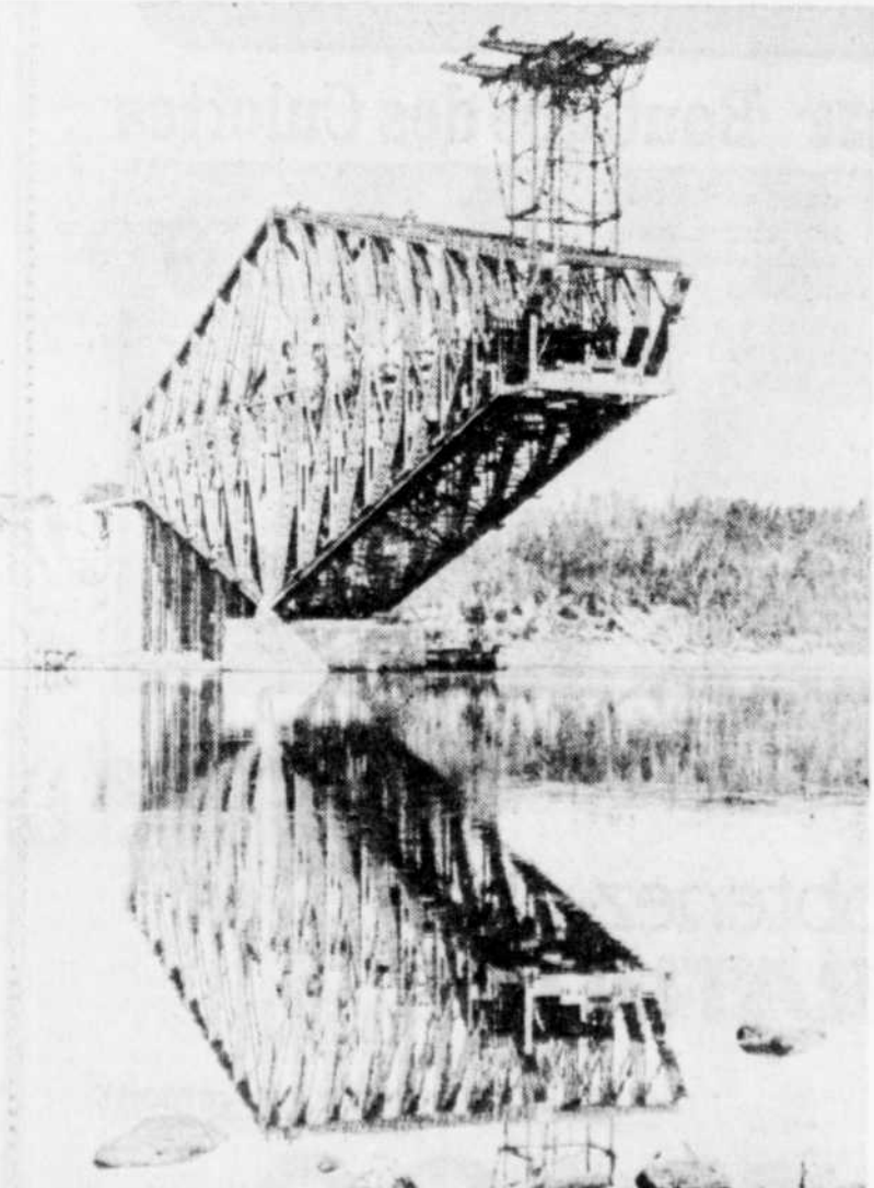
À l'automne 1915, cette photo du bras nord du pont de Québec montre comment la deuxième version était déjà plus solide que la première structure (photos de droite).
