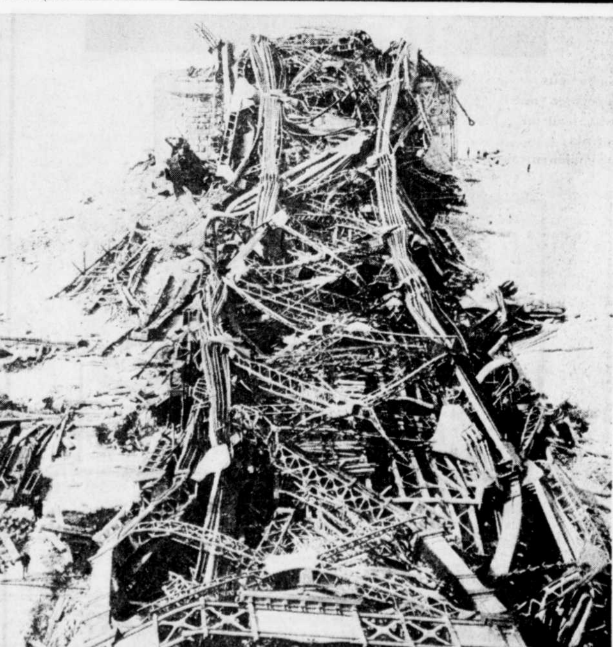
La première version du pont de Québec, sur la rive sud, était moins large (67 pieds au lieu de 88) et plus mince d'acier. Elle s'effondra en 1907, tuant 76 personnes.
