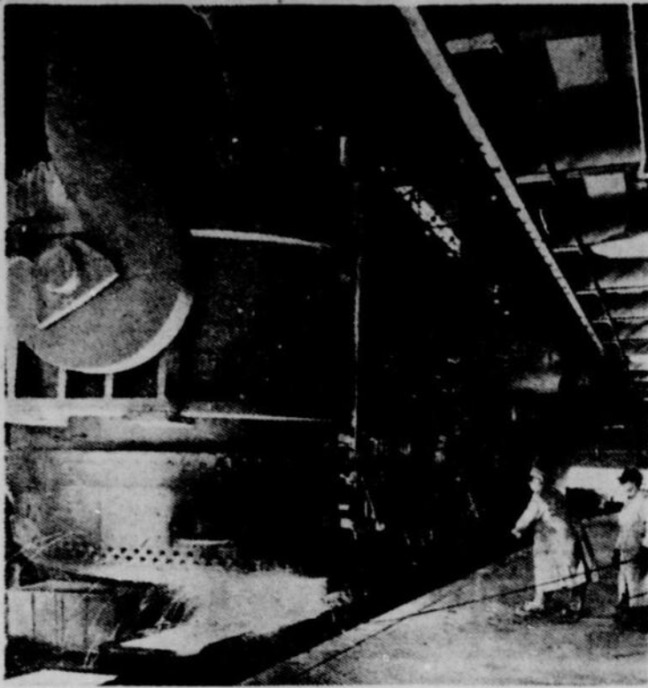
Pour la première opération de dégrossissage dans une aciérie comme la STELCO, on utilise un laminoir de blooming (ci-dessus) qui transforme le lingot en brame ou en bloom.
