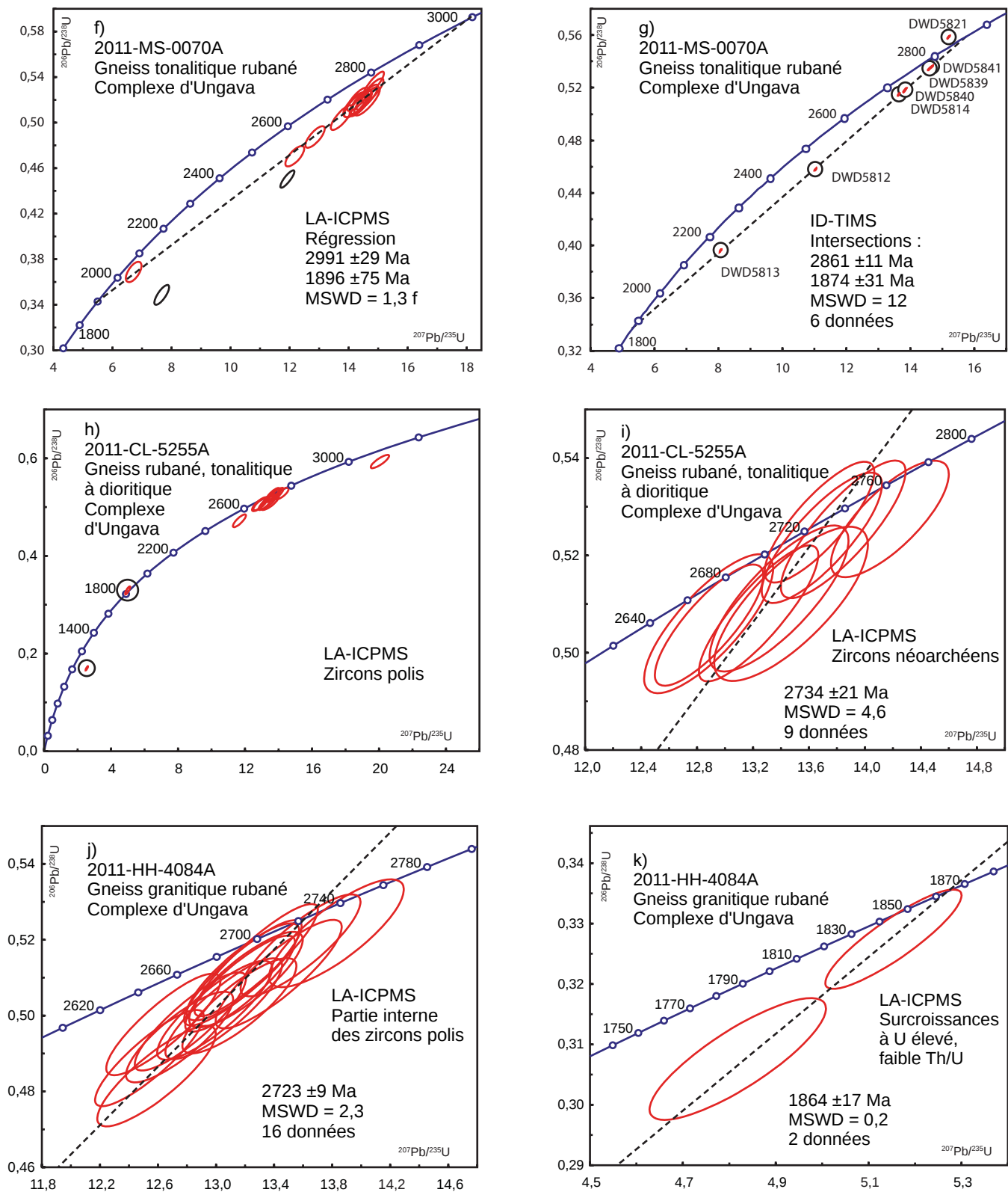
FIGURE 7 (SUITE) – Diagrammes concordia (7f à 7k) des analyses des zircons et des monazites pour les échantillons en provenance du secteur de Kuujuaq et de la baie d'Ungava effectuées par la méthode LA-ICPMS et ID-TIMS. Les résultats analytiques sont présentés aux tableaux 2 et 3. MSWD = Mean Squared Weighted Deviates.
