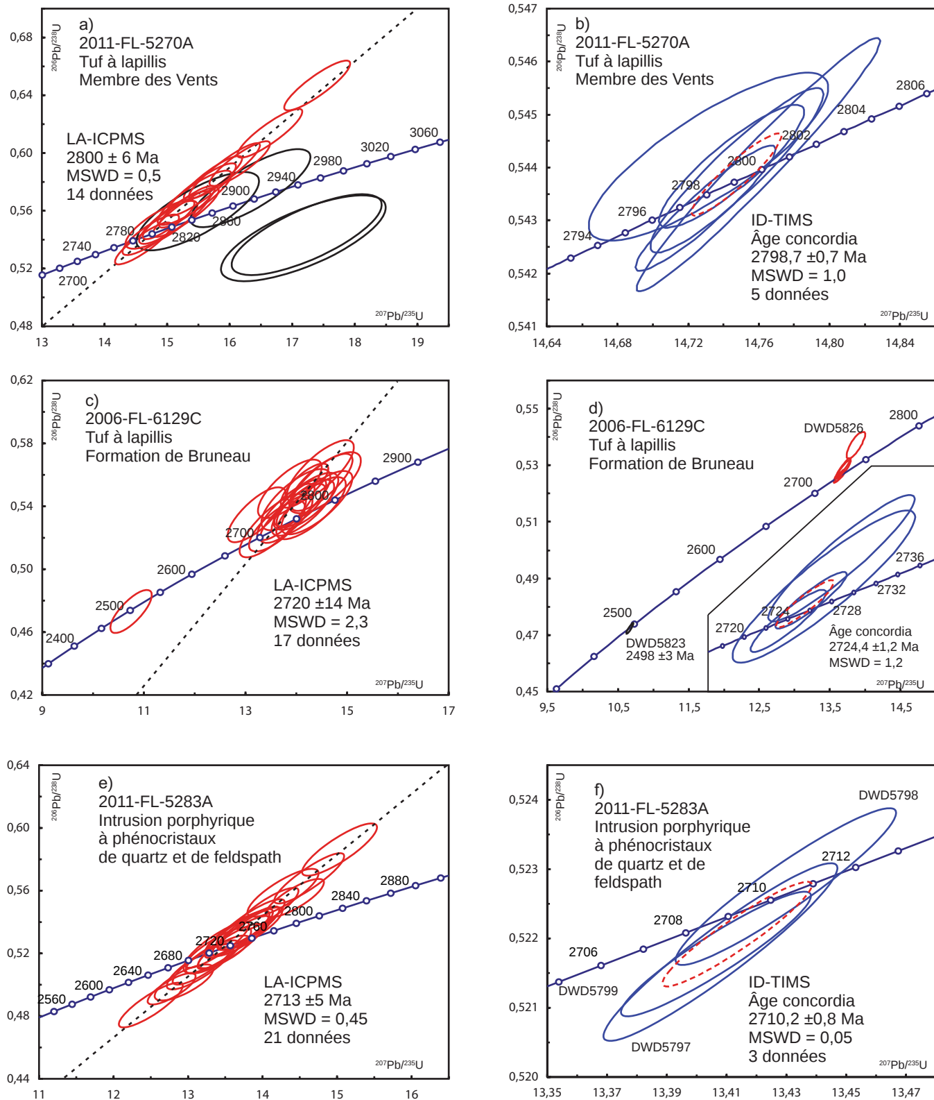
FIGURE 9 – Diagrammes concordia des analyses de zircons pour les échantillons en provenance de Chibougamau-Chapais et de Matagami effectuées par la méthode LA-ICPMS et ID-TIMS. Les résultats analytiques sont présentés aux tableaux 2 et 3. MSWD = Mean Squared Weighted Deviates.
