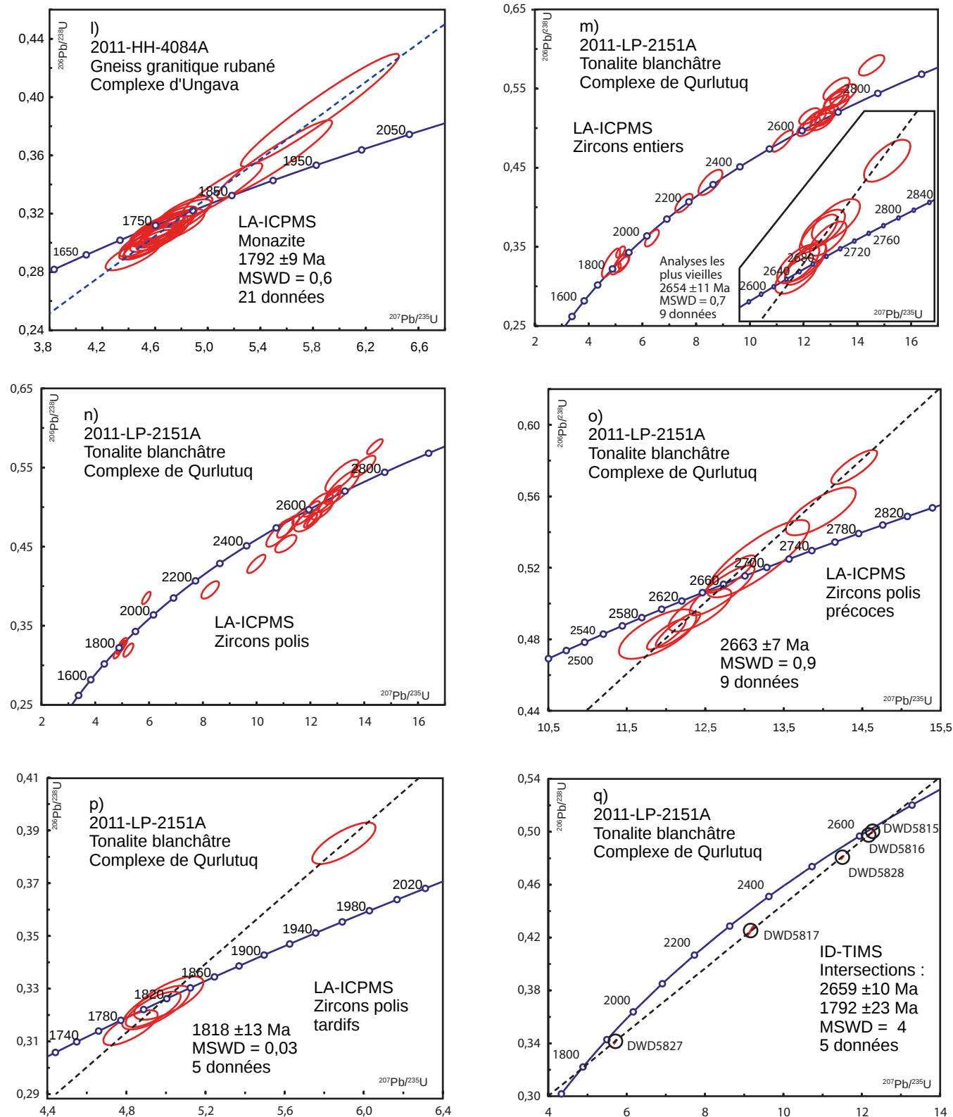
FIGURE 7 (SUITE) – Diagrammes concordia (7l à 7q) des analyses des zircons et des monazites pour les échantillons en provenance du secteur de Kuujuaq et de la baie d'Ungava effectuées par la méthode LA-ICPMS et ID-TIMS. Les résultats analytiques sont présentés aux tableaux 2 et 3. MSWD = Mean Squared Weighted Deviates.
