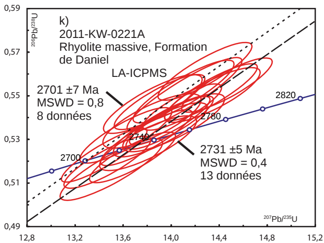
FIGURE 9 (SUITE) – Diagrammes concordia des analyses de zircons pour les échantillons en provenance de Chibougamau-Chapais et de Matagami effectuées par la méthode LA-ICPMS et ID-TIMS. Les résultats analytiques sont présentés aux tableaux 2 et 3. MSWD = Mean Squared Weighted Deviates.
