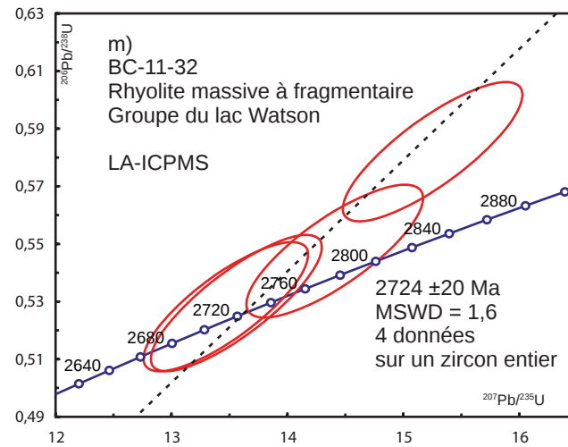
FIGURE 9 (SUITE ET FIN) – Diagramme concordia des analyses de zircons pour les échantillons en provenance de Chibougamau-Chapais et de Matagami effectuées par la méthode LA-ICPMS et ID-TIMS. Les résultats analytiques sont présentés aux tableaux 2 et 3. MSWD = Mean Squared Weighted Deviates .
