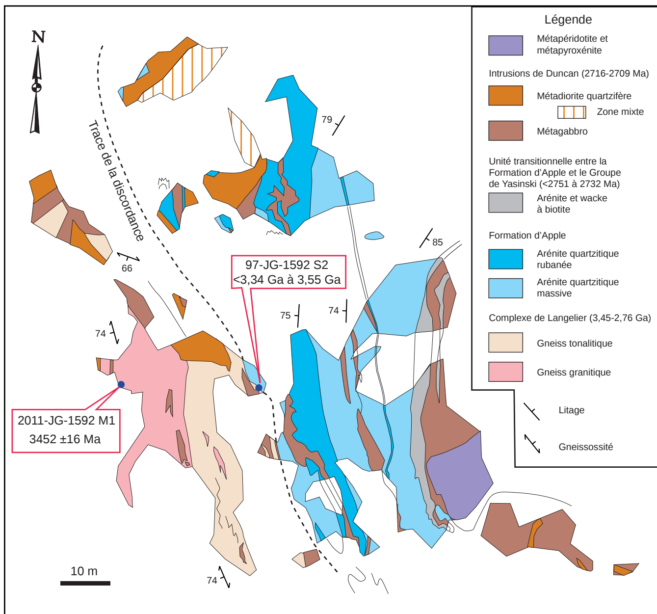
FIGURE 4 – Carte détaillée de l’affleurement 1997-JG-1592 (SNRC 33F04) où est illustrée la localisation des échantillons prélevés pour la datation d’un gneiss du Complexe de Langelier et des zircons détritiques dans l’arénite quartzitique de la Formation d’Apple. Cet affleurement contient la plus vieille roche de la Baie-James et le deuxième secteur des plus vieilles roches du Québec.
