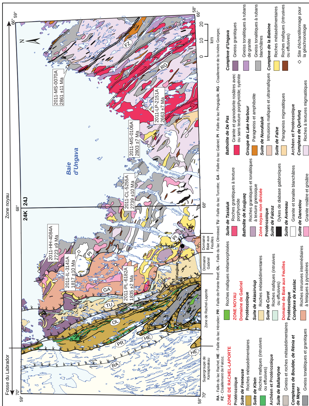
FIGURE 2 – Géologie simplifiée de la région de Kuujuaq et de la baie d'Ungava et localisation des sites d'échantillonnage de géochronologie.
