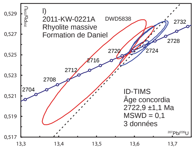
FIGURE 9 (SUITE) – Diagrammes concordia des analyses de zircons pour les échantillons en provenance de Chibougamau-Chapais et de Matagami effectuées par la méthode LA-ICPMS et ID-TIMS. Les résultats analytiques sont présentés aux tableaux 2 et 3. MSWD = Mean Squared Weighted Deviates.
