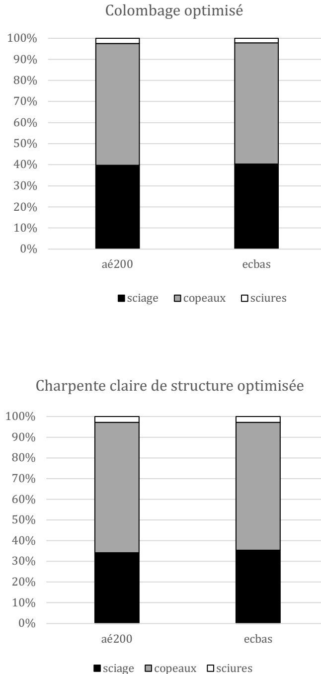
Figure 5 : Proportion des sciages, des copeaux et des sciures par modalité d'éclaircie et par procédé de débitage. Aucune différence significative (ANOVA, p > 0,05 ) entre les modalités d'éclaircie pour les sciages, copeaux et sciures pour chacun des procédés de débitage ni entre les procédés de débitage pour une même modalité d'éclaircie
