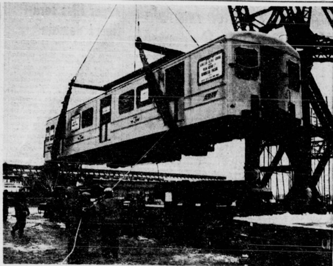
VOICI L'UN DES QUATRE NOUVEAUX WAGONS DESTINÉS AU MÉTRO DE TORONTO et qui ont été chargés hier, dans le port de Montréal, sur des wagons plates-formes spéciaux du Canadien National. Au contraire des 100 wagons en acier déjà commandés par la Toronto Transportation Commission, ces quatre nouvelles unités ont une superstructure en aluminium qui les rend beaucoup moins lourdes que les wagons actuellement en usage. Ils pèsent cinquante tonnes de moins que les wagons en acier.
