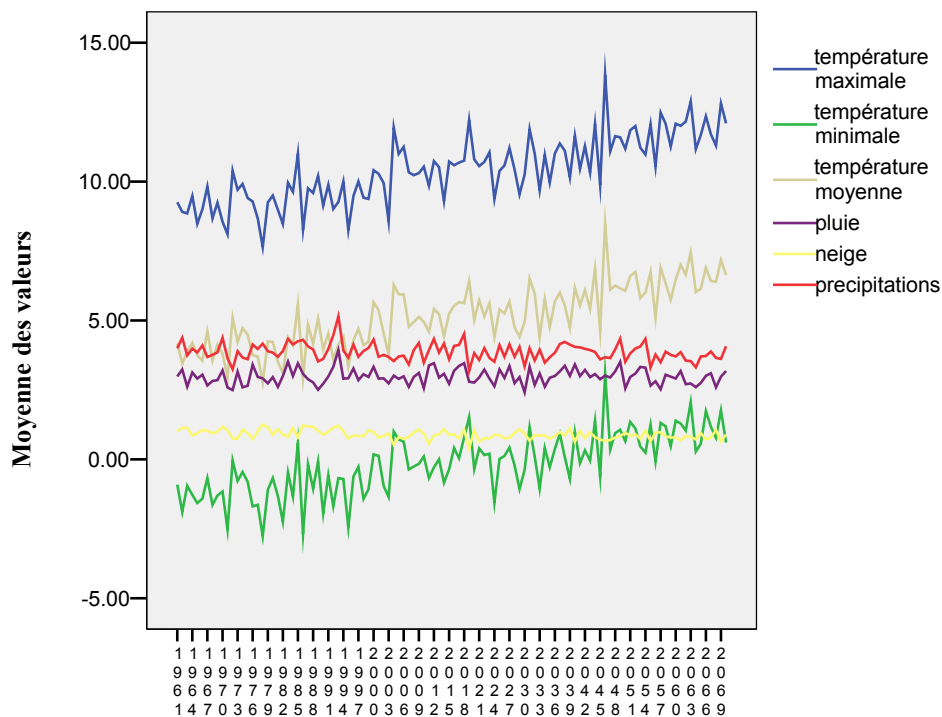
Figure 2.37. Températures (°C), précipitations (mm), pluie (mm) et neige (cm) selon modèle HadCM3 scénario B, après Downscaling, station Québec.
