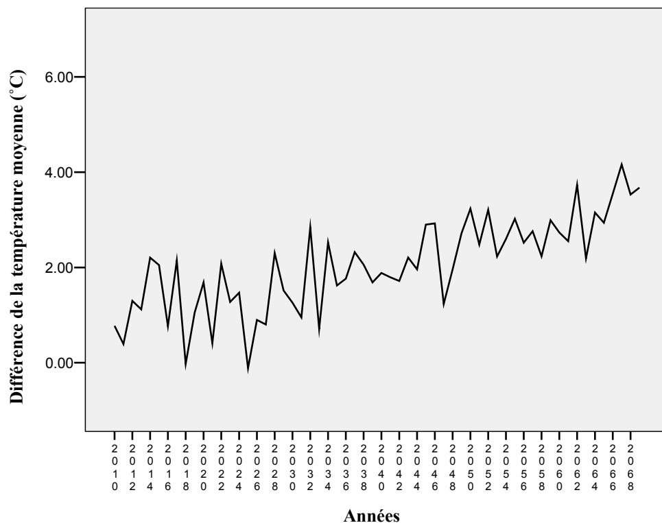
FIGURE 2.13. Fluctuations de la température moyenne journalière future par rapport à la période contrôle 1961-1990 simulée par le modèle CGCM1, après downscaling, station St-Hippolyte.
