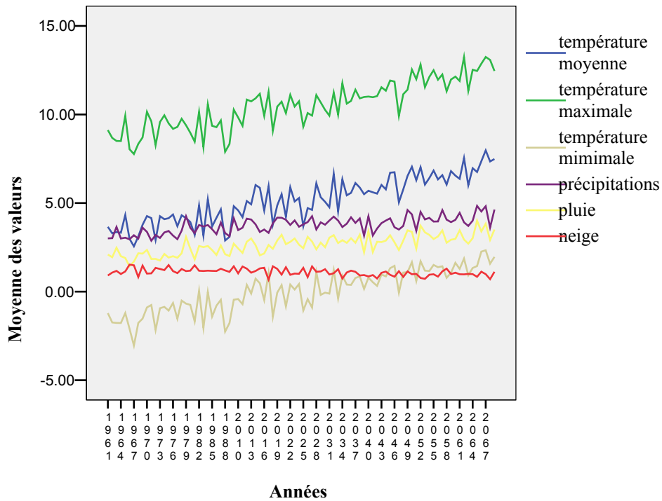
Figure 2.24. Températures (°C), précipitations (mm), pluie (mm) et neige (cm) selon modèle CGCM1, après Downscaling, station Sutton.
