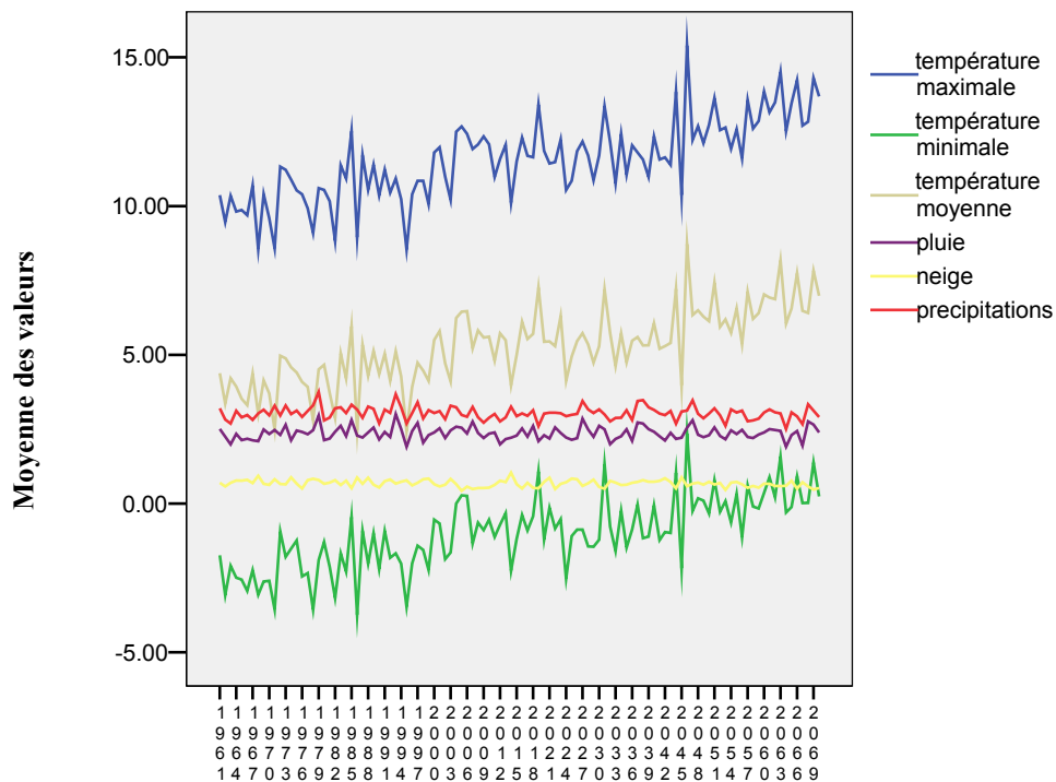
Figure 2.38. Températures (°C), précipitations (mm), pluie (mm) et neige (cm) selon modèle HadCM3 scénario B, après Downscaling, station Sherbrooke.
