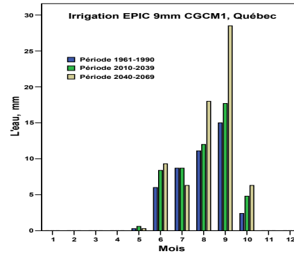
Figure 5.22 Irrigation préconisée (critère de 9mm), Québec, CGCM1, 3 périodes
