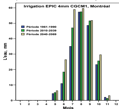
Figure 5.10 Irrigation préconisée (critère de 4mm), Montréal, CGCM1, 3 périodes
