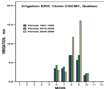
Figure 5.23 Irrigation préconisée (critère de 13mm), Québec, CGCM1, 3 périodes
