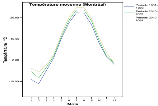
Figure 5.7 La température moyenne à Montréal pendant trois périodes (données du CGCM1 après “downscaling”)
