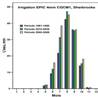
Figure 5.16 Irrigation préconisée (critère de 4mm), Sherbrooke, CGCM1, 3 périodes
