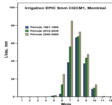
Figure 5.11 Irrigation préconisée (critère de 9mm), Montréal, CGCM1, 3 périodes
