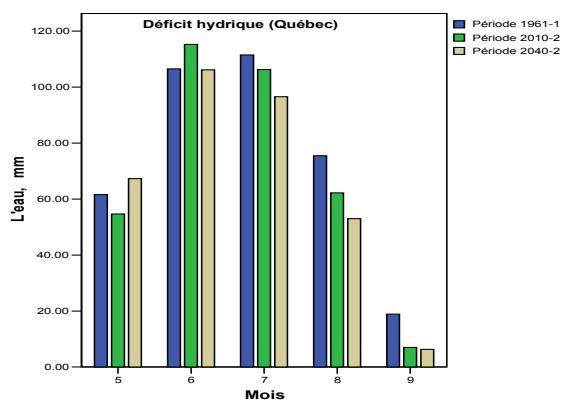
Figure 5.21 Déficit hydrique à Québec
