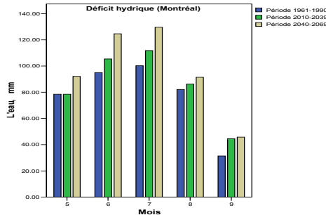
Figure 5.9 Déficit hydrique à Montréal
