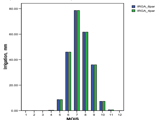
Figure 5.5. Irrigation préconisée, critère de 10 mm, avec 4 (IRGA_4par) et 6 paramètres (IRGA_6par) pour la région de Montréal, 1961-90 (données observées)
