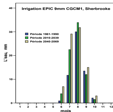
Figure 5.17 Irrigation préconisée (critère de 9mm), Sherbrooke, CGCM1, 3 périodes
