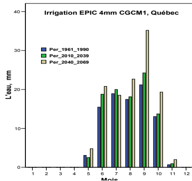
Figure 5.21 Irrigation préconisée (critère de 4mm), Québec, CGCM1, 3 périodes
