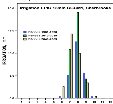
Figure 5.18 Irrigation préconisée (critère de 13mm), Sherbrooke, CGCM1, 3 périodes
