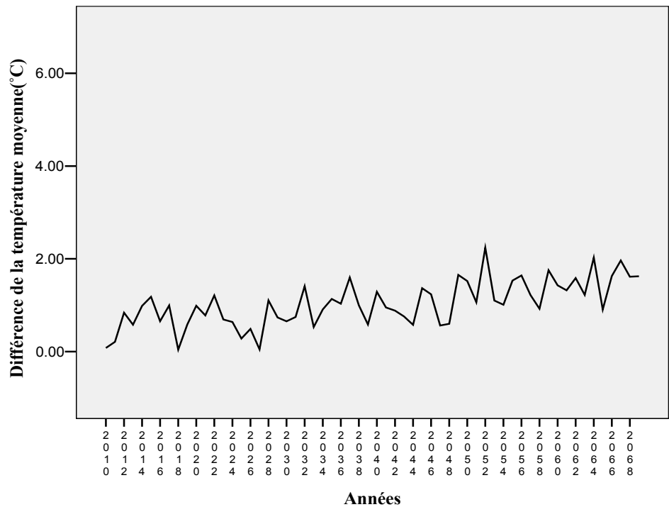
FIGURE 2.1. Fluctuations de la température moyenne journalière future par rapport à la période contrôle 1961-1990 simulée par le modèle CGCM1, après Downscaling, station Grand Fonds.
