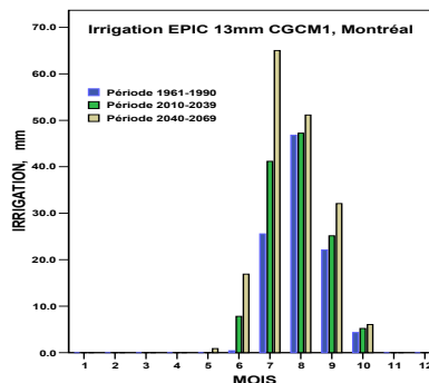
Figure 5.12 Irrigation préconisée (critère de 13mm), Montréal, CGCM1, 3 périodes
