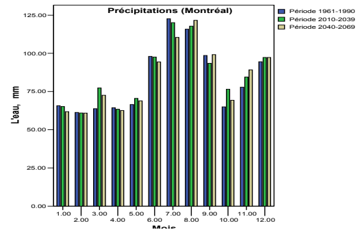
Figure 5.8 Les précipitations à Montréal pendant trois périodes (données du CGCM1 après “downscaling”)
