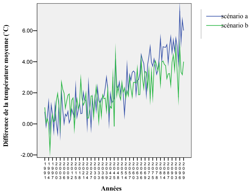
FIGURE 2.14. Fluctuations de la température moyenne journalière future par rapport à la période contrôle 1961-1990 simulée par le modèle HadCM3, après downscaling, station St-Hippolyte.
