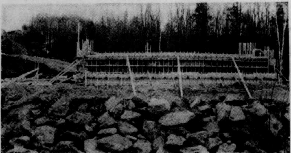
Les travaux pour l'érection d'un pont qui traversera la rivière Niger près de Ayer's Cliff vont bon train. C'est la firme Couillard Construction Ltée de Coaticook qui exécute les travaux de l'ordre de $326,073. Ce pont permettra d'unir la route (ancienne route 50) menant à Coaticook par Ayer's Cliff. Cette photo a été prise de la route 5 qui traverse l'ancienne route 50 aujourd'hui portant le numéro 141. Ce montant comprend également de l'asphalte et l'érection d'un câble rigide. (Photo La Tribune, Studio Pépin, Rock Island)
