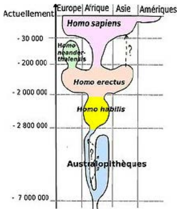
Schéma montrant l'évolution simplifiée des hominidés à travers le temps (dates approximatives en années) et leur distribution sur la planète [6].
