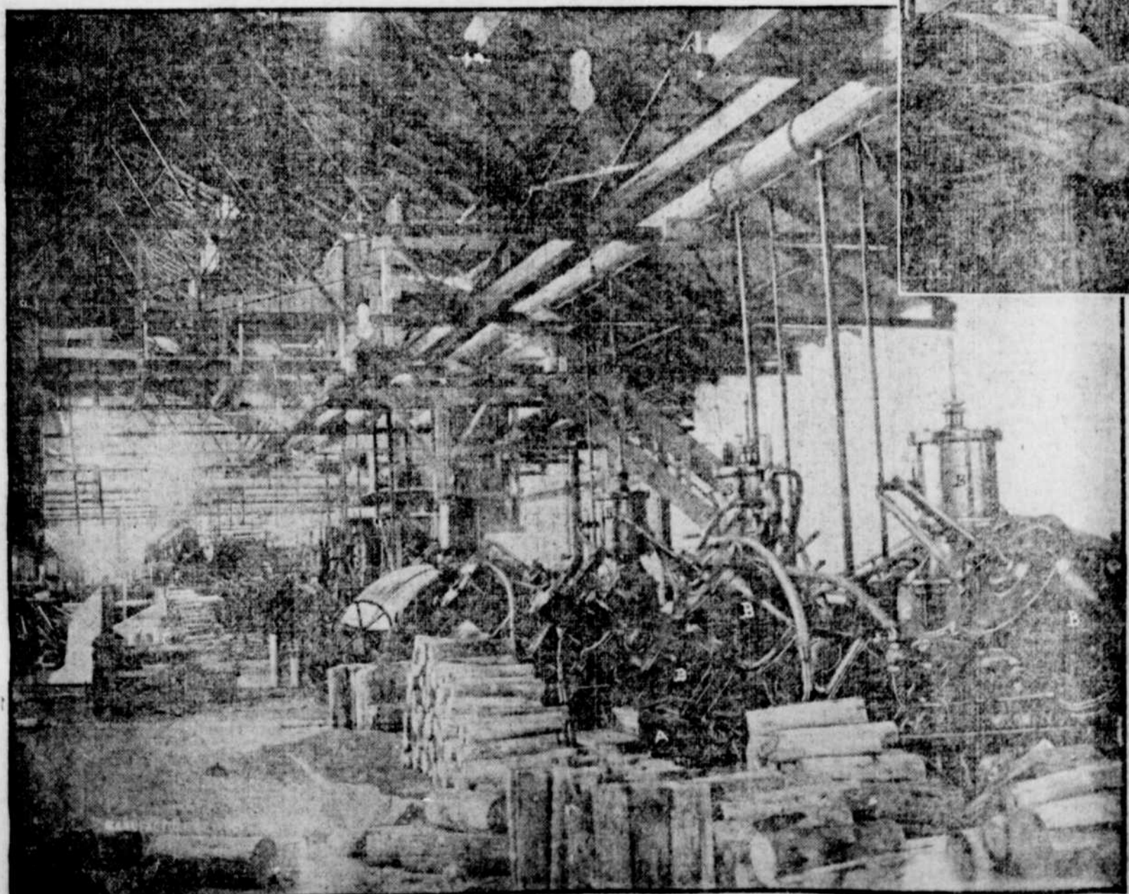
VUE DES RÉSERVOIRS À FONDS DE TAMIS OÙ CIR- CULE LA PÂTE DE PULPE, ET OÙ À L'IMPÉRIUM LES CYLINDRES D'AGGLOMÉRATION.
