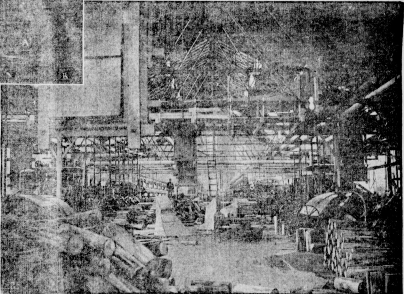
VUE GÉNÉRALE DE L'INTÉRIEUR DE LA PULPERIE NEUVE TOUTE CONSTRUITE EN PIERRE ET EN FER. Les BATTERIES DE DÉFIBREUSES DANS LA PULPERIE NEUVE. LE BOIS DE PULPE ÉCORCÉ PRÉALABLE- MENT, EST RÉDUIT EN PÂTE.
