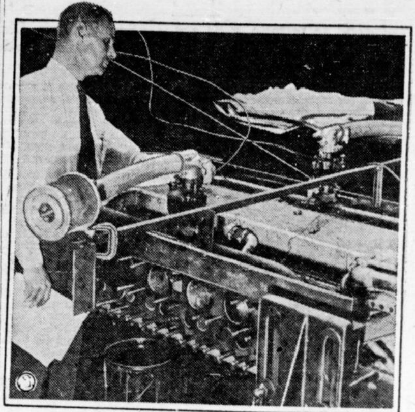
L'ingénieur H. C. Church, de Cleveland, Ohio, près du moteur 12 cylindres White à travail horizontal qu'il a imaginé et construit. Ce moteur servira pour les autobus. Sa construction permet de le placer au centre de la grosse voiture. Il n'a que 16 pouces de hauteur, et ne prend pas beaucoup de place.
