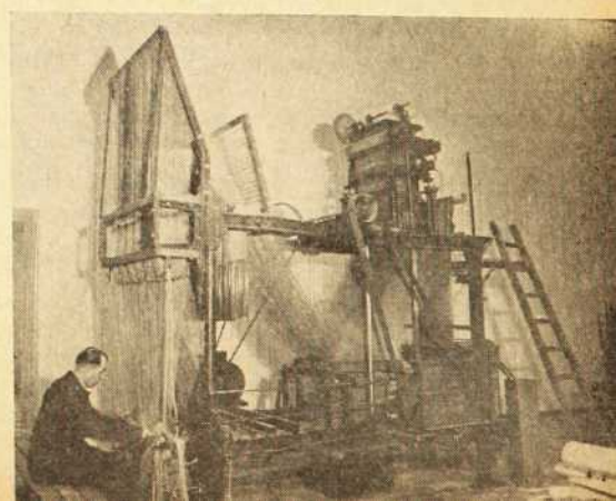
Autre machine de tissage en usage dans les soieries de Lyon, les plus célèbres du monde entier. Ph. S.F.T.
