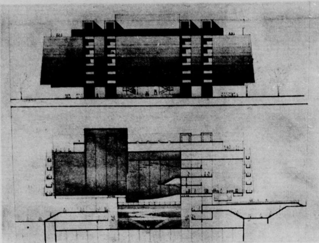
En haut, extérieur du Pavillon vu de face. En bas, coupe latérale de l'édifice : on distingue les coursives de circulation au pourtour intérieur ; à l'extrémité droite, l'entrée principale de la façade et les escaliers qui mènent au foyer du théâtre.
