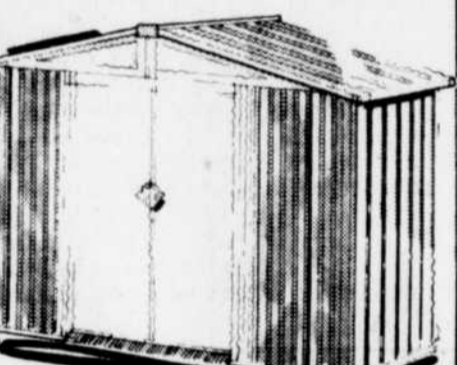
Remise "Steelcolor" Remise fabriquée en acier émaille blanc et vert. Dimensions extérieures: 96" x 85" x 71" de hauteur. Superficie de 51' cu. 12888 chac.
