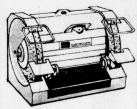
Touret Shopmate 5" 3.2 amp. et moteur à 3500 t. m. à l'épreuve du grillage. 2 meules de 5" x 1/2" x 1/2". =2601. 3754 chac.
