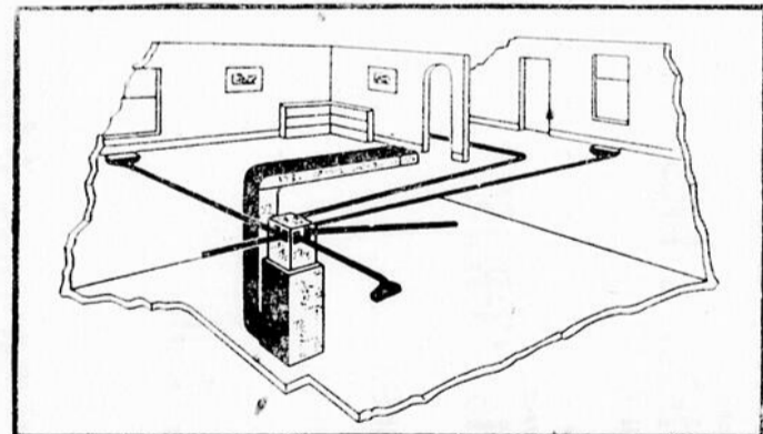
Système périmétrique de climatisation en hiver avec petits conduits individuels
