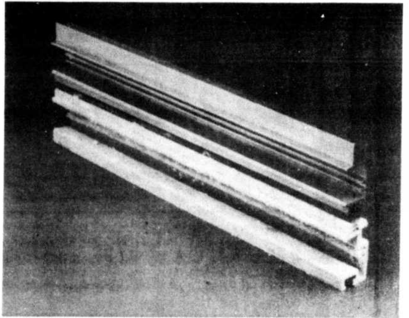
Cette coupe du cadre en aluminium d'une fenêtre moderne démontre comment l'isolant agit efficacement comme barrière thermique dans la transmission de la chaleur. La partie extérieure est gelée alors que la partie intérieure est chaude.
