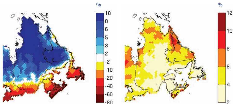
Figure 3 : Changement moyen (gauche) (2041-2070 vs 1961-1990) et écart-type des changements (droite) de l'équivalent en eau de la neige cumulée au sol en mars. Les changements sont estimés d'après un ensemble de 5 simulations du MRCC pilotées par 5 membres différents du modèle couplé climatique global (MCCG3) selon le scénario d'émissions de gaz à effet de serre A2 (SRES A2).
