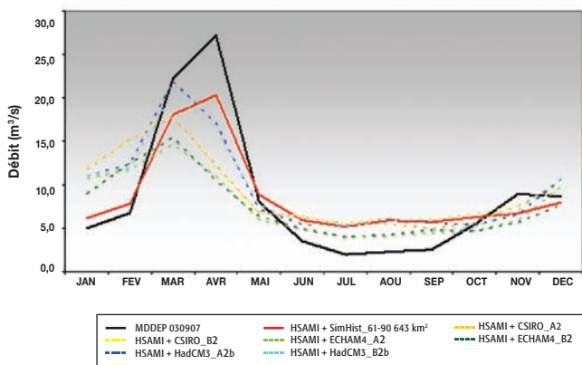
Rivière : Des Anglais / Station : 030907 / Régime :NAT / Superficie : 643 km 2 HSAMI - Période historique (1961-90) et années 2040-69 en CC
