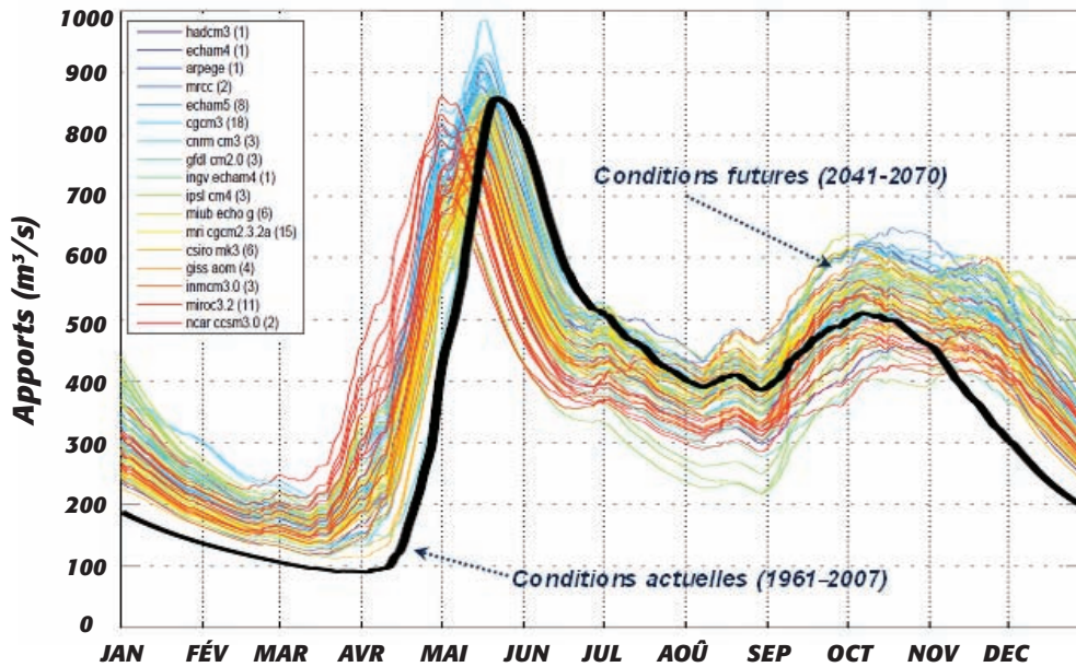
Figure 16 : Hydrogrammes moyens reconstitués et futurs pour chacune des 90 simulations — bassins versants du Nord québécois (Roy et al. , 2008b).
