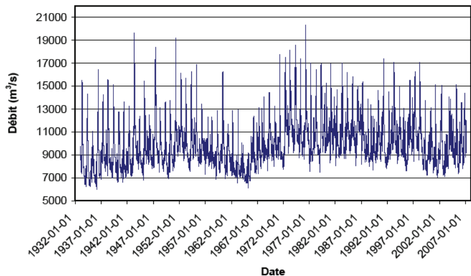
Figure 20 : Débit du Saint-Laurent à Sorel, 1 er janvier 1932 au 1 er janvier 2007 (Morin et Bouchard, 2000 ; J.-F. Cantin, communication personnelle).
