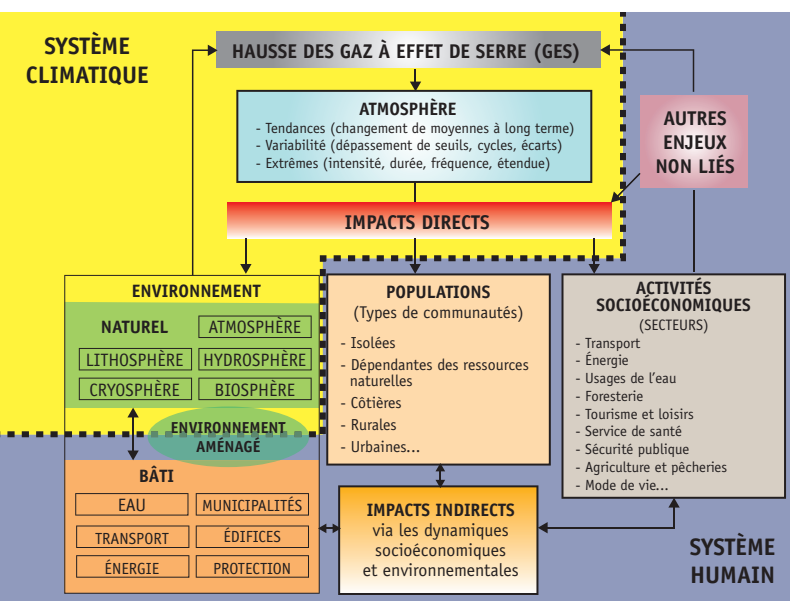
Figure 8 : Impacts directs et indirects du climat, de sa variabilité et de ses extrêmes sur l'environnement naturel et bâti, les populations et les activités socioéconomiques.
