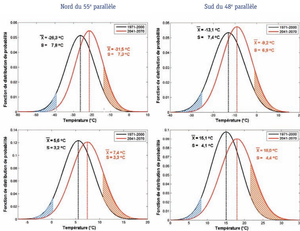
Figure 5 : Distributions hivernales (DJF) (haut) et estivales (JJA) (bas) des températures quotidiennes moyennes simulées en climat actuel (1971-2000) et projetées dans le futur (2041-2070) par un ensemble de 5 simulations MRCC4.2.3 pilotées par 5 différents membres de MCG3 sur la base du scénario A2. Les zones hachurées représentent les 10 e et 90 e percentiles basés sur le climat actuel. X̄ et S réfèrent respectivement à la moyenne et à l'écart-type de la distribution.
