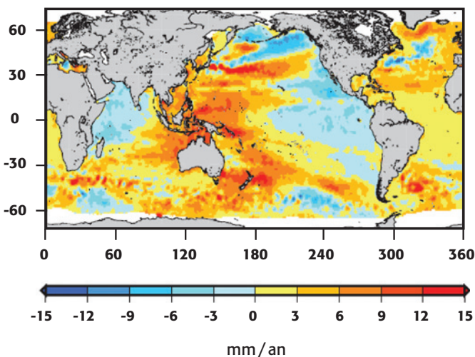
Figure 12 : Distribution géographique des tendances linéaires à court terme pour le niveau moyen de la mer, dans la période 1993-2003 (mm/an), sur la base des données altimétriques du satellite Topex-Poséidon (GIEC, 2007a).
