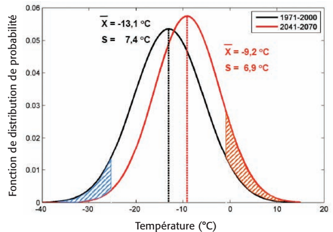
Figure 18 : Distribution hivernale (DJF) des températures quotidiennes moyennes au sud du 48° parallèle simulées en climat actuel (1971-2000) et projetées dans le futur (2041-2070) par un ensemble de 5 simulations MRCC4.2.3 pilotées par 5 différents membres de MCG3 sur la base du scénario A2. Les zones hachurées représentent les 10 e et 90 e percentiles basés sur le climat actuel. \bar{X} et S réfèrent respectivement à la moyenne et à l'écart-type de la distribution.
