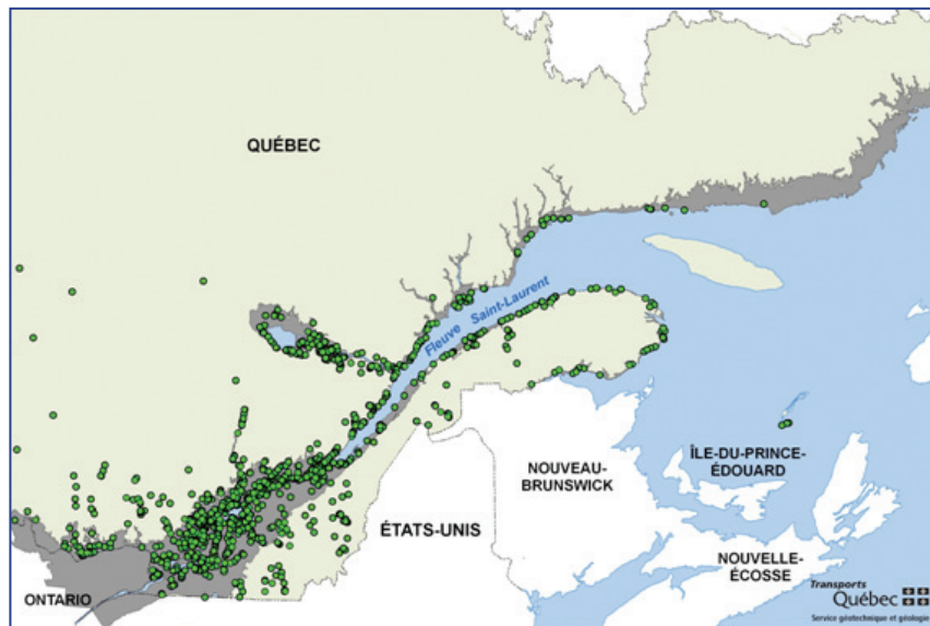
Figure 28 : Inventaire des demandes d'intervention pour des glissements de terrain au Québec, entre 1972 et 2005 (carte fournie par le MTQ, communication personnelle). La zone en gris foncé montre les limites de l'invasion marine postglaciaire à dépôts argileux.
