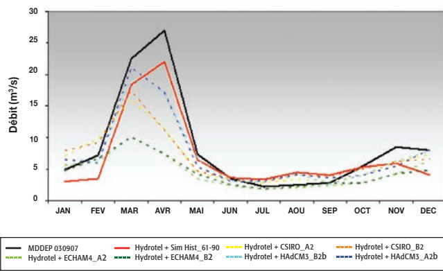
Rivière : Des Anglais / Station : 030907 / Régime :NAT / Superficie : 643 km 2 Hydrotel+ParPrev - Période historique (1961-90) et années 2040-69 en CC
