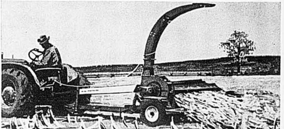
Elle filamente et étend les pieds de blé d'Inde, les tiges de coton, les rameaux taillés dans le verger; elle chaume le riz, taille l'herbe des prés!
