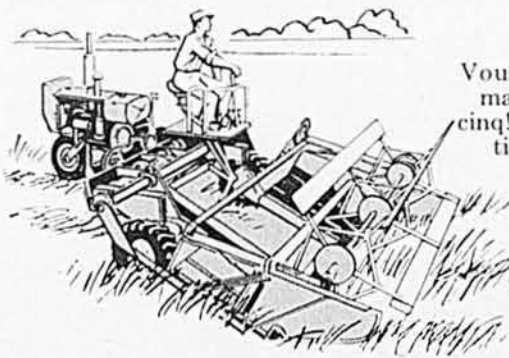
Andaineuse Automotrice McCormick No 163
