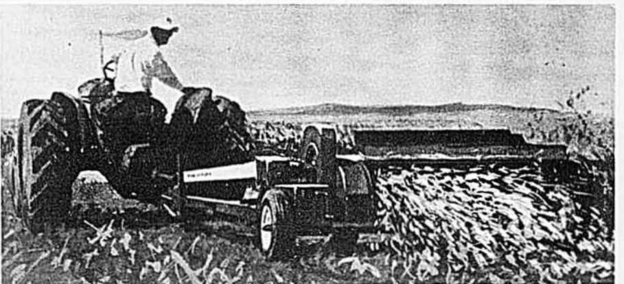
La nouvelle filamenteuse de récolte "31" fait rapidement toutes sortes de travaux de nettoyage à votre ferme.
