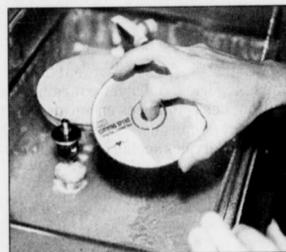
Des gouttes d'eau tombent régulièrement sur la ponceuse pour empêcher le disque de chauffer.
