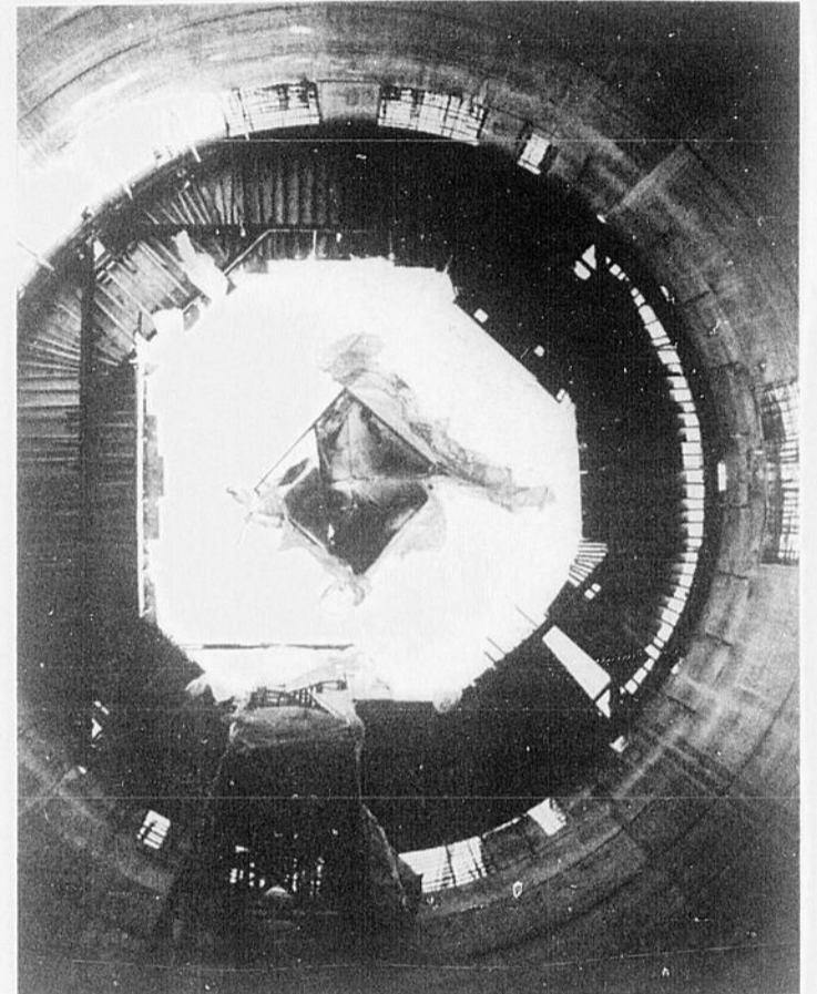
UNE VUE SAISSANTE, du fond d'un des silos, du type de plate-forme qui s'est effondrée au chantier du Mont Wright. Les quatre coins du grand cadre d'acier que l'on distingue, surmonté de planches n'étaient retenus que par une simple soudure...
