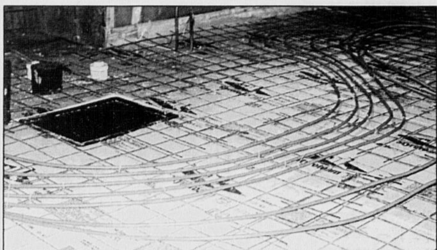
Après avoir isolé le plancher de ce sous-sol, on coulera une dalle de béton sur les tuyaux de chauffage radiant hydraulique.
