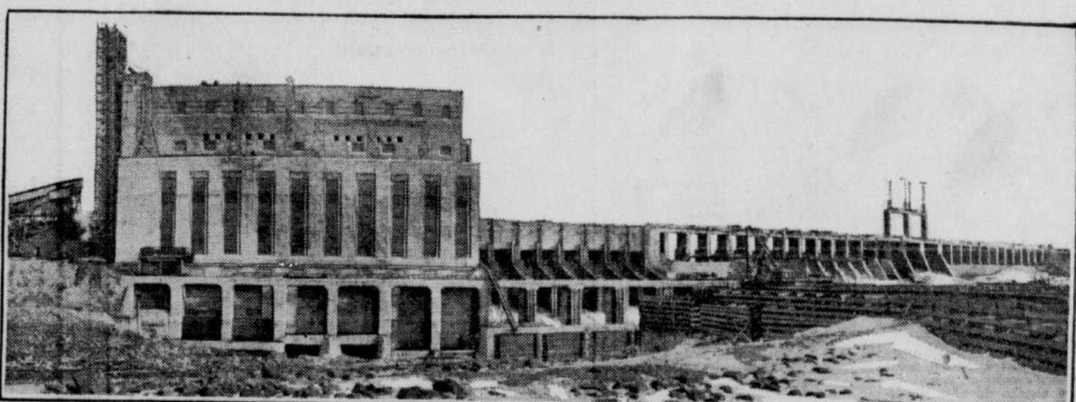
Centrale génératrice des Sept Seurs de la Northwestern Power Company Limited, sur la rivière Winnipeg. Puissance 225,000 HP. Par ses services de génie et de construction, la Power Corporation of Canada Limited, a coopéré à la construction de cette usine dont deux unités sont maintenant terminées.
