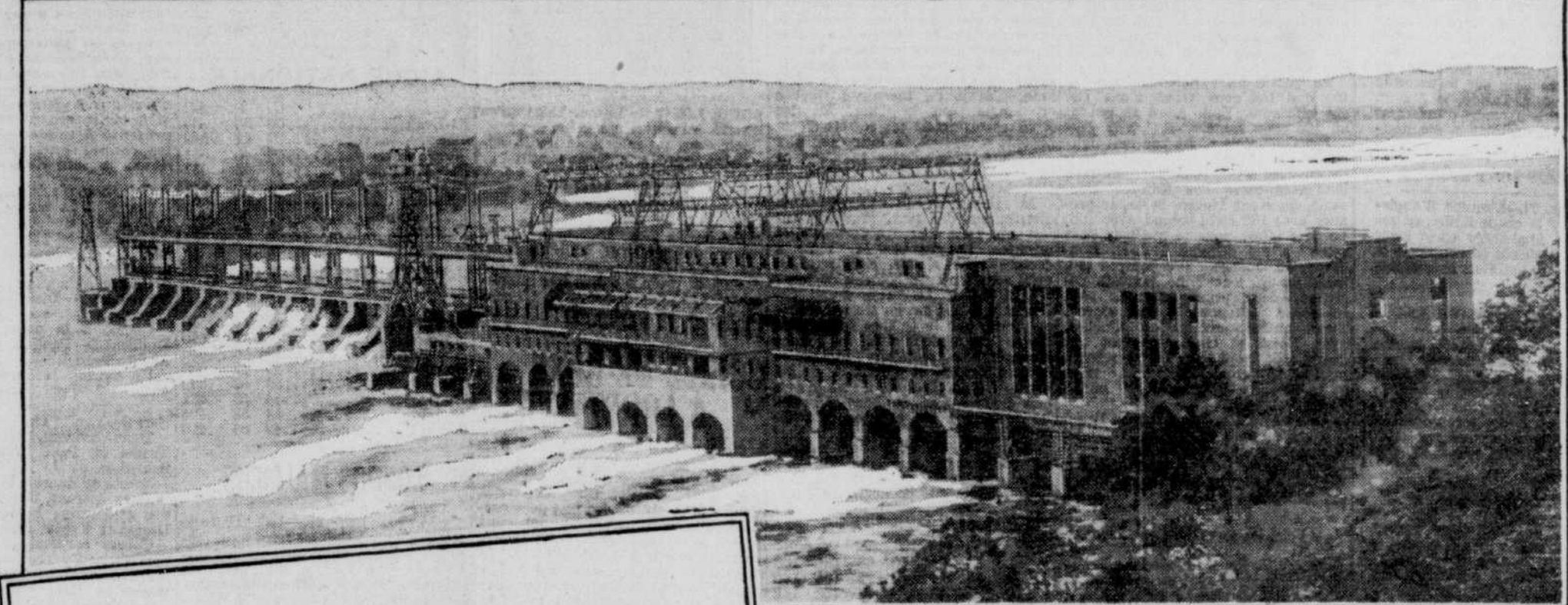
Centrale génératrice sur la rivière des Prairies de la Montreal Island Power Company Limited, puissance maximum 78,000 HP. Plans et construction de cette centrale par la Power Corporation of Canada Limited.
