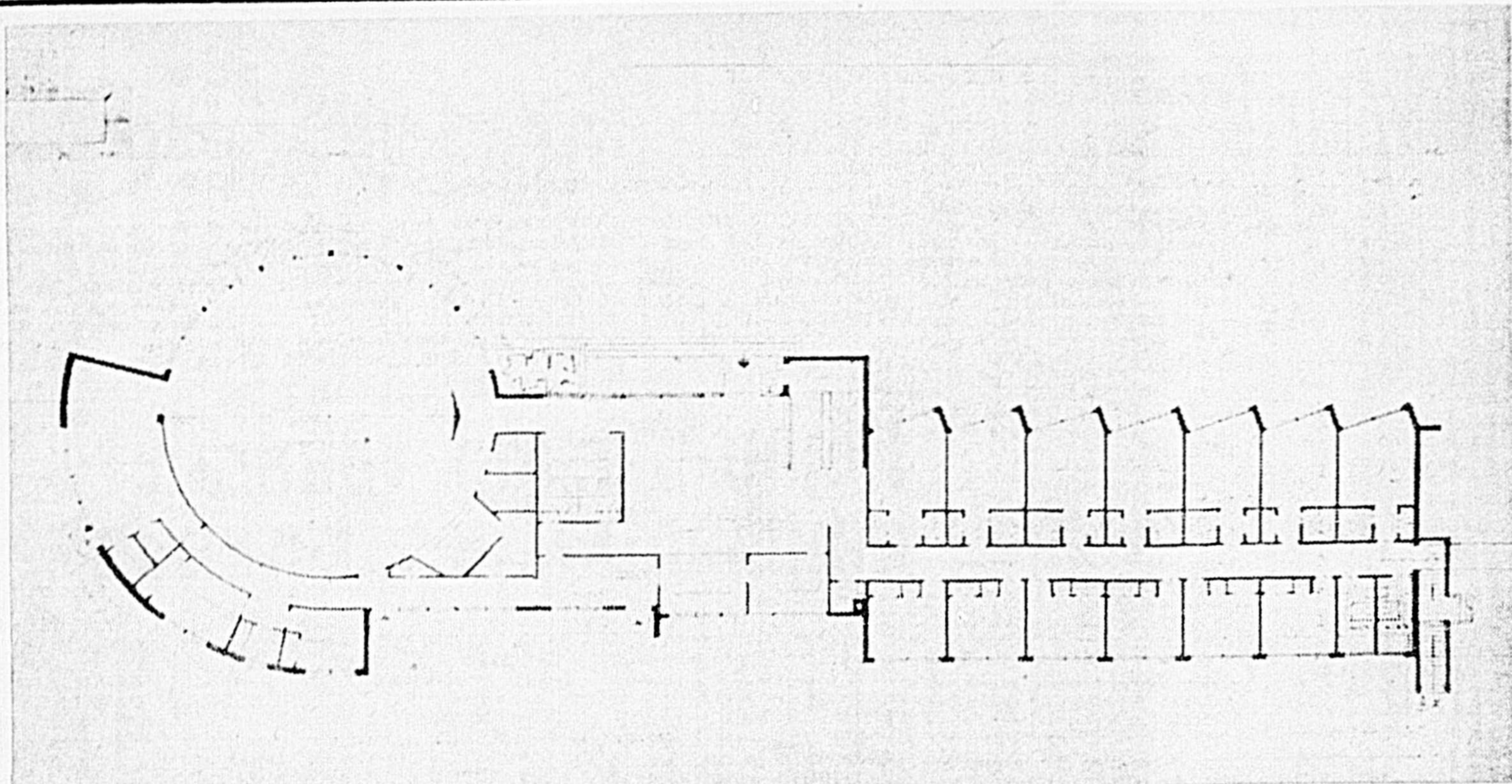
PLAN DE L'HOTEL DE L'ISLE-MALIGNE: le Manoir-du-Rocher, dessiné par M. Maurice Gravel, architecte de Chicoutimi. L'hôtel peut se subdiviser en trois sections principales. A gauche du plan: deux étages de chambres et un cocktail-lounge en sous-sol. Surface totale: 4,716 pieds carrés, volume global: 100,610 pieds cubes. Au centre du plan: l'administration et le hall d'entrée avec sur la "chambre". Surface totale: 1,500 pieds carrés. Volume global: 28,000 pieds cubes. A droite du plan: section salle à manger et salle de réception avec dépendance, cuisine, dépôt, bar, chambres pour personnel résident. Surface totale: 400 pieds carrés. Volume global: 40,000 pieds cubes.
