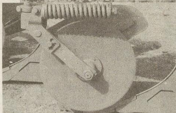
COUTRES CIRCULAIRES À RESSORT
