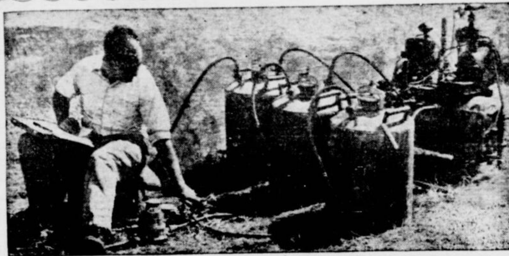
Réservoirs contenant le liquide extincteur sous pression. Les tuyaux servent à relier les réservoirs avec la pompe à incendie.
