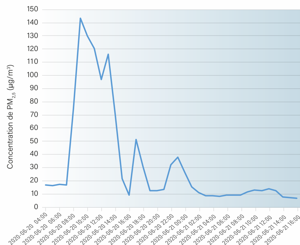
Concentrations horaires de PM 2.5 entre le 20 et le 21 juin 2020 à la station Pémonca
