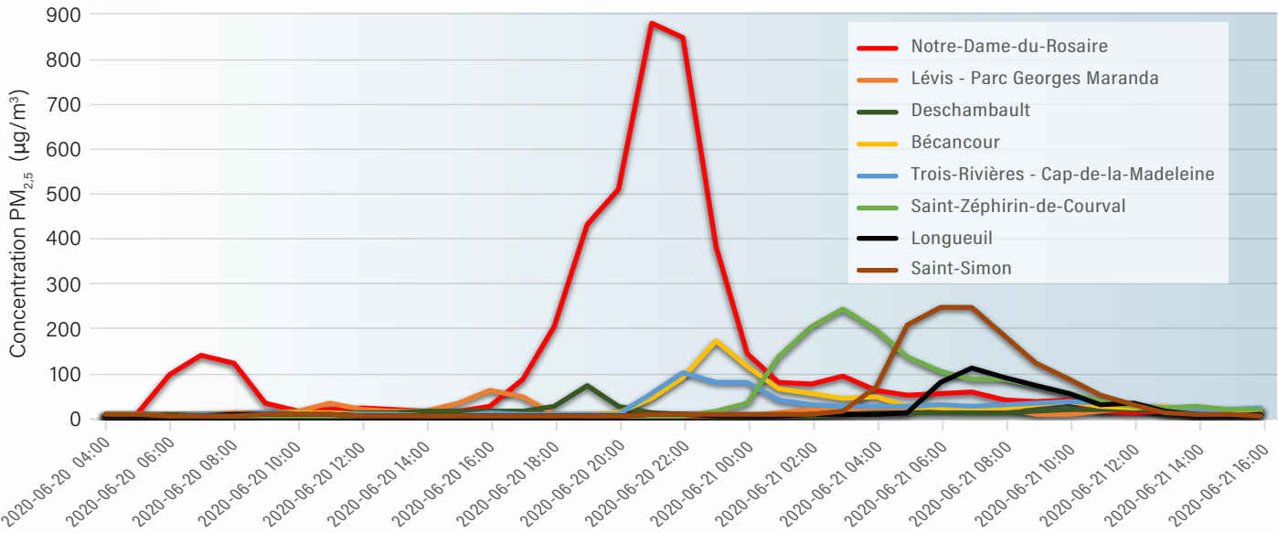
Concentrations horaires de PM_{2,5} entre le 20 et le 21 juin 2020
