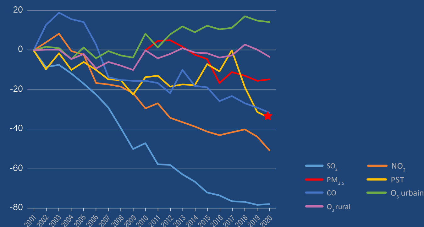
Pourcentage de variation des concentrations de contaminants dans l'air au Québec
