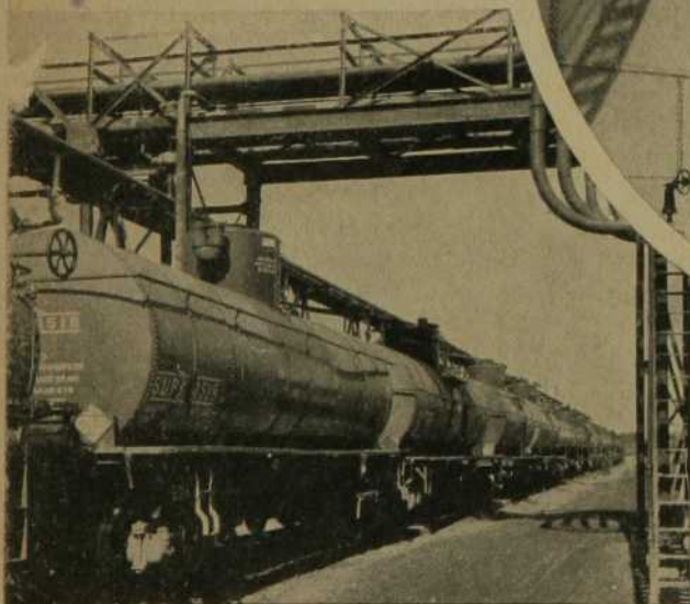
LE CHARGEMENT DES WAGONS... Les produits pétroliers sont chargés dans les wagons-réservoirs au moyen de gros conduits suspendus. Les wagons quittent ensuite la raffinerie de l'Imperial Oil pour aller porter leurs précieux chargements dans toutes les parties du pays. Les produits de l'Imperial Oil, vendus dans tout le Canada, sont toujours de qualité uniforme.
