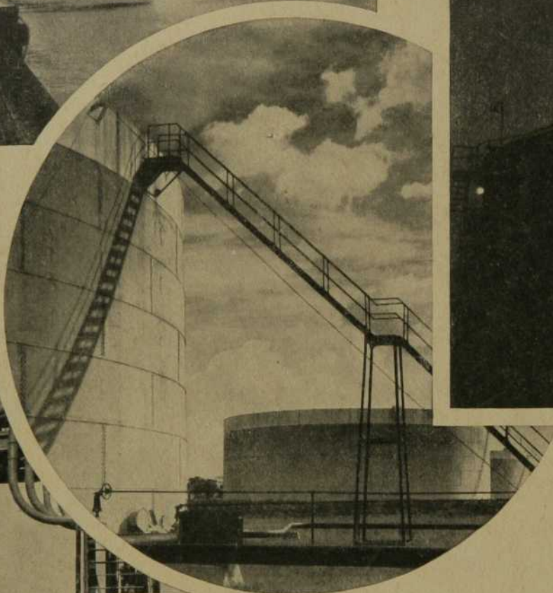
POUR L'EMMAGASINAGE DE L'HUILE... (à gauche) Nous voyons ici quelques-uns des immenses réservoirs qui servent à l'emmagasinement de l'huile brute et des produits raffinés à l'établissement de Sarnia, Ontario. Chacun de ces réservoirs a une capacité de 3,000,000 de gallons. La capacité totale des réservoirs de l'Imperial Oil à cet endroit est de 150,000,000 de gallons. C'est une réserve nécessaire pour protéger les consommateurs en cas de disette.
