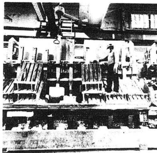
Changement d'anode sur une cuve précurtée
