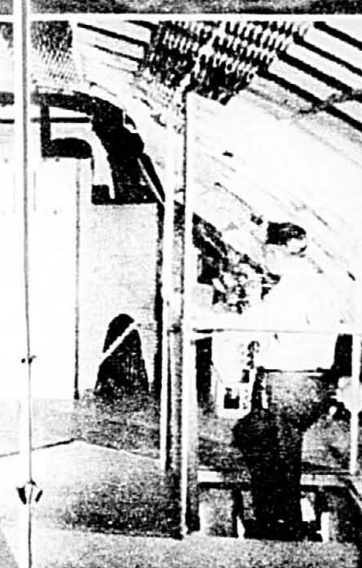
Le démontage du hangar primitif va bon train (extrême gauche), tandis qu'aux carrefours le fuselage de l'hydravion a la priorité (au centre). Cf-contre: le vaste poste de pilotage auquel on accède par un escalier en colimaçon (debout, au fond: Howard Hughes). A droite: deux remorqueurs maintiennent le Spruce Goose au milieu du chenal; construction cantiléver du nouveau hangar.
