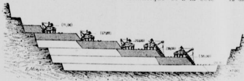
Schéma du travail des excavateurs dans les chantiers de la Culebra. (Les chiffres indiquent l'altitude des gradins successifs.)
