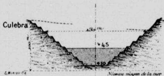
Coupe du bief de partage à la Culebra. (La partie hachurée indique les terres restant à enlever.)
