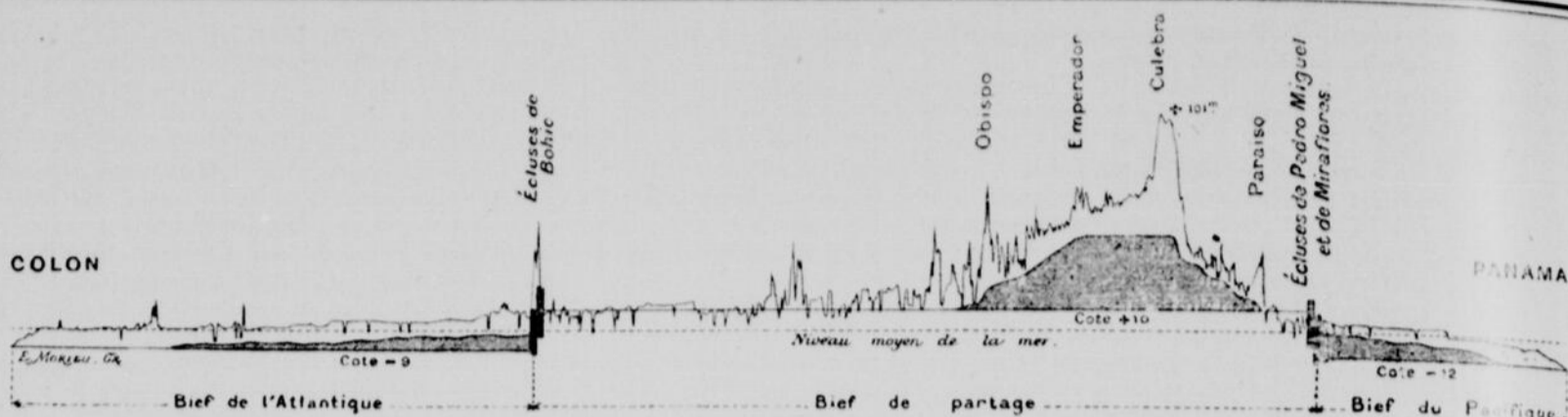
Coupe suivant l'axe du canal. — (Les parties hachurées indiquent les principaux cubes de terre restant à enlever.)
