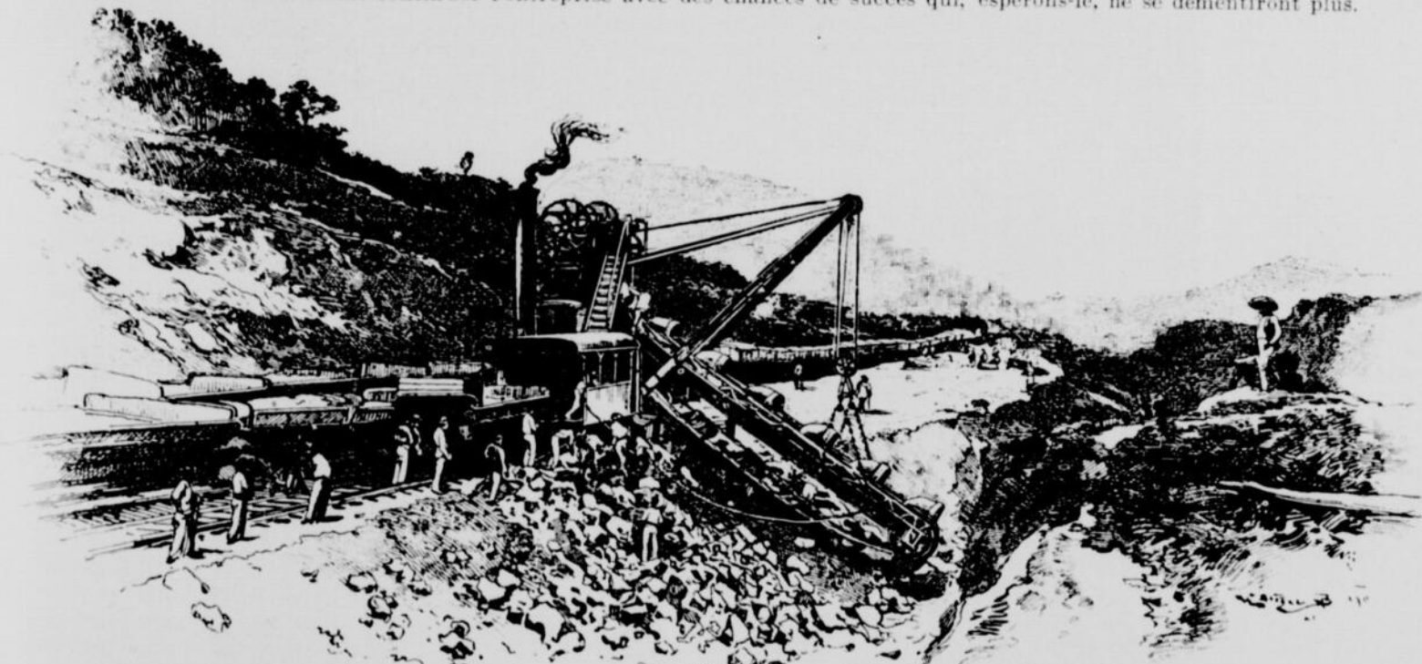
Un excavateur à Cucaracha
