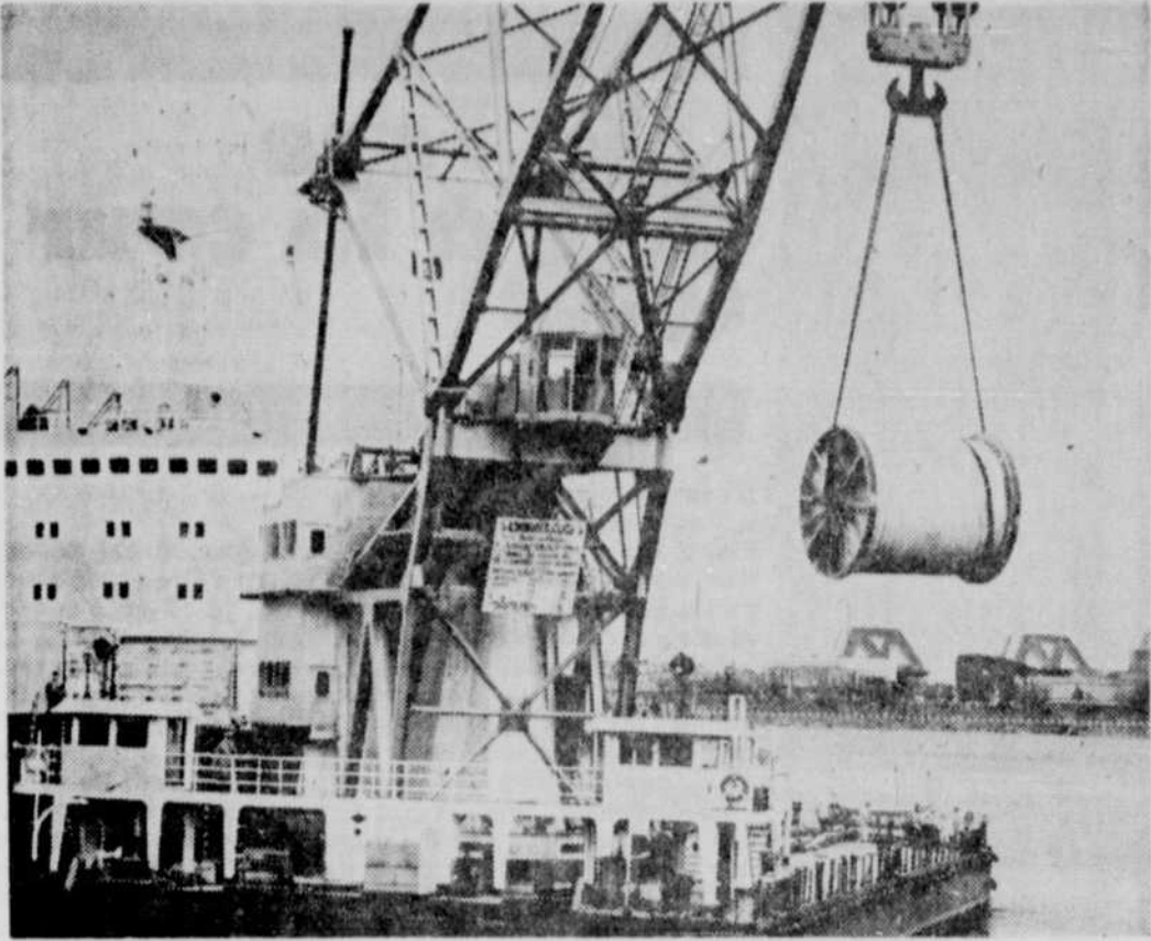
Le câble téléphonique sous-marin le plus long et le plus lourd jamais fabriqué par la Northern Electric a récemment quitté le port de Montréal à bord d'un cargo à destination de la Turquie. Il a été fabriqué à Lachine, pèse 75 tonnes et mesure 11,300 pieds. Dans le cadre d'un contrat de 5 ans d'une valeur de $24.5 millions, plus de 110 tours de câbles téléphoniques ont été expédiés vers la Turquie cette année.
