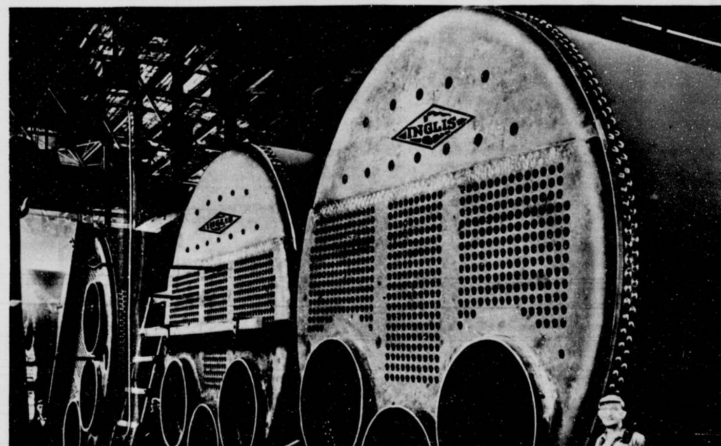
AU COMMANDEMENT "AVANT, TOUTES!" ces chaudières de navires "Scotch" accomplissent leur travail avec une aisance miraculeuse. Elles sont construites par INGLIS pour service sur les navires de la Patrouille navale canadienne. Le capitaine et l'équipage peuvent compter sur la force motrice indéfectible développée et la vitesse et la mobilité que fournissent ces énormes chaudières.
