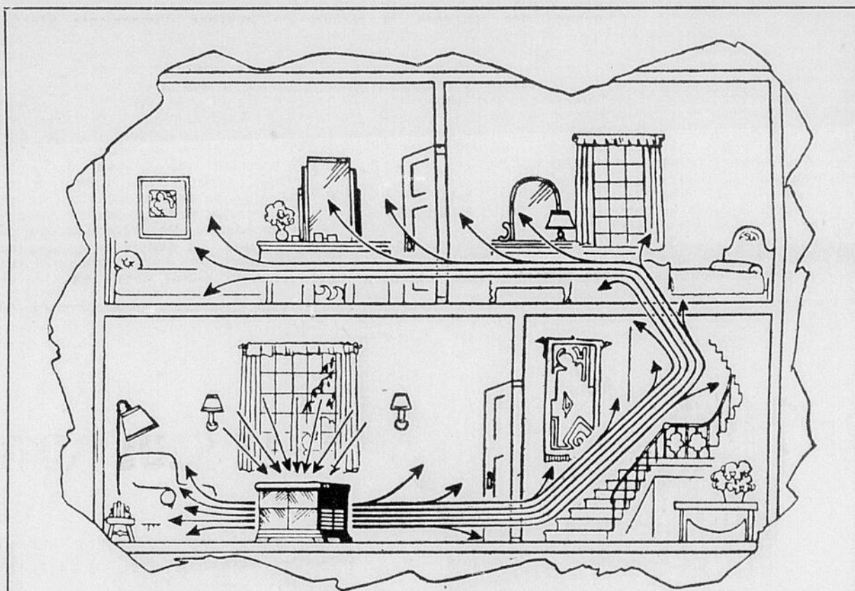
Ce dessin vous fait voir approximativement comment l'air circule dans la maison ordinaire. Dans une maison à deux étages, même les coins les plus éloignés bénéficient de l'air en circulation — de l'air mobile qui circule dans un vaste espace et remplace l'air sec et contaminé.
