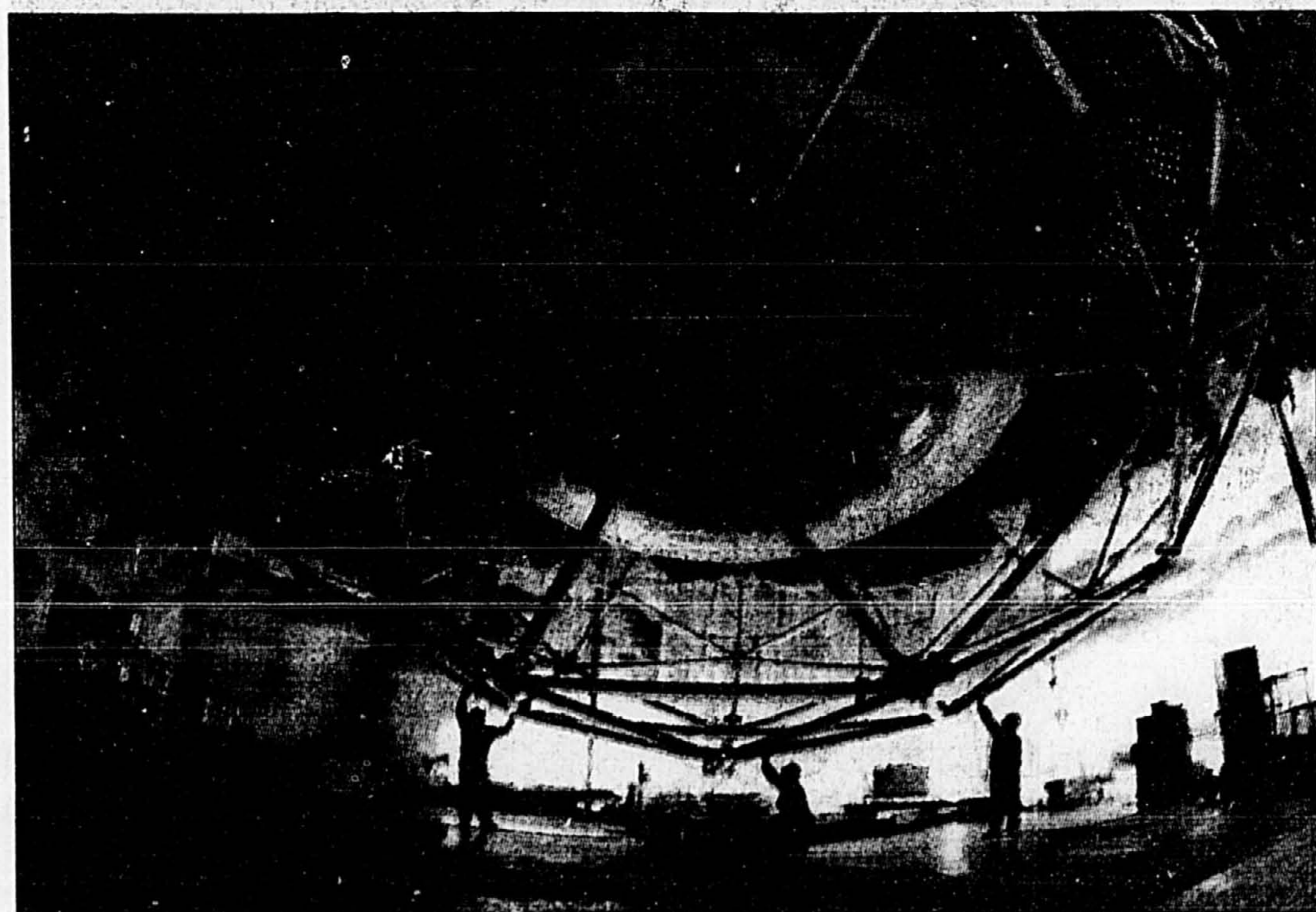
L'Observatoire de neutrinos de Sudbury est situé au fond d'une mine. Celle-ci abrite une sphère de 12 mètres de diamètre contenant de l'eau lourde, autour de laquelle a été assemblée une autre sphère, géodésique, parsemée de 10 000 photodétecteurs qui guetteront les rayons gamma caractéristiques des collisions des neutrinos avec les molécules d'eau lourde.
