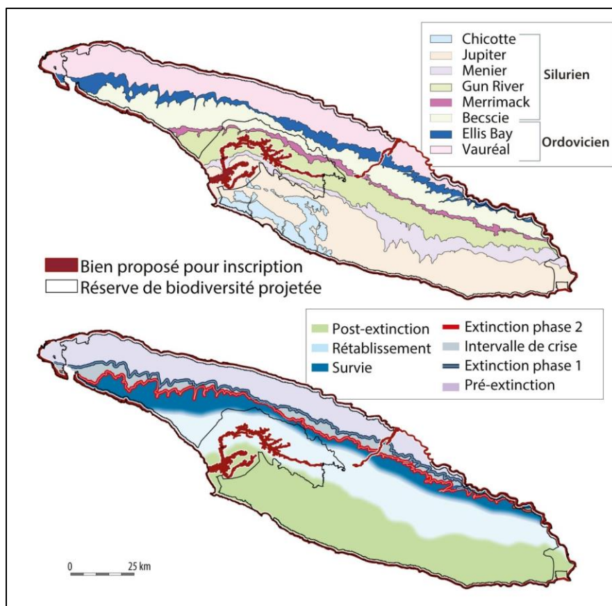
Figure 12. Recouplement de la RBP d'Anticosti avec les strates géologiques et leur correspondance avec les événements de la première extinction de masse du vivant
