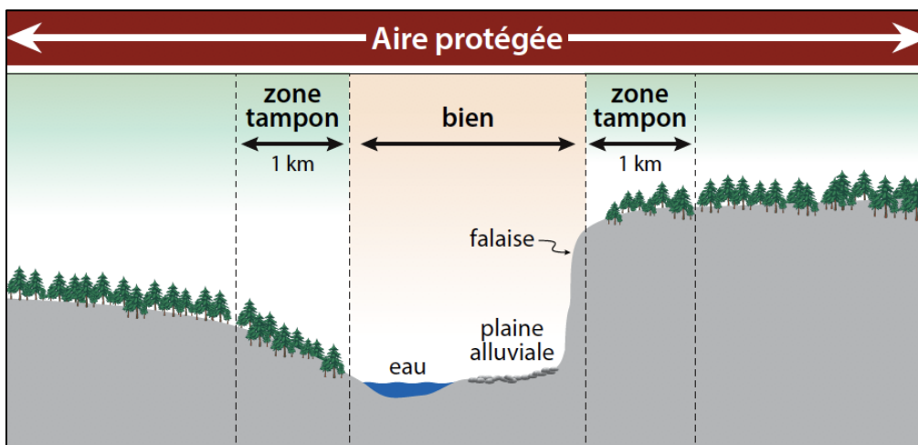
Figure 10. Schéma d'une coupe transversale du bassin fluvial montrant que les limites de la RBP englobent le bien, une zone tampon d'un kilomètre de chaque côté du bien ainsi qu'une zone supplémentaire au-delà des zones tampons pour protéger la majorité du bassin versant
