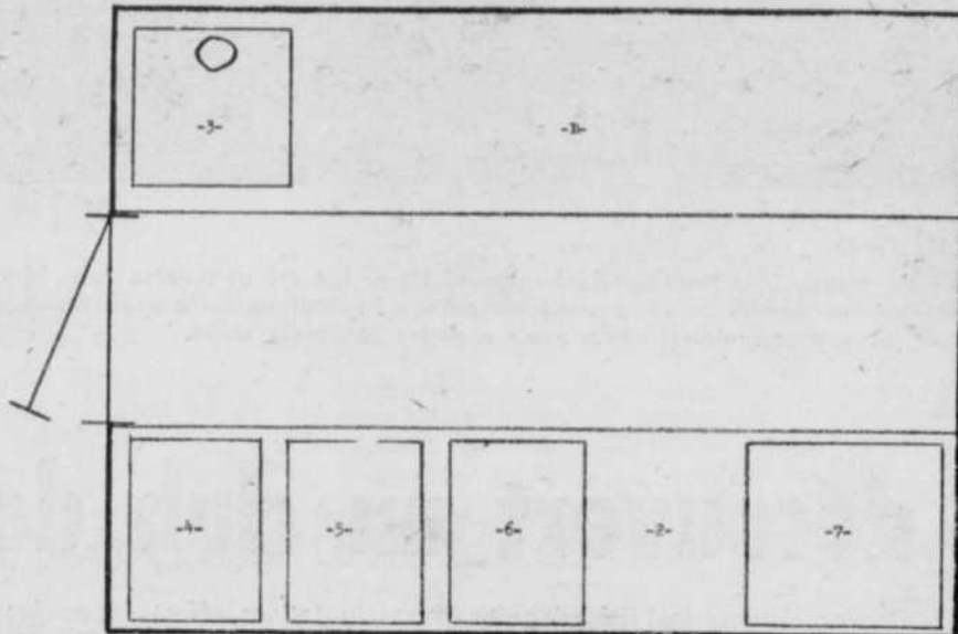
Idéalement toujours, un labo fonctionnel peut être aménagé comme ceci. En — 1 —, la partie sèche (8'x2') sur laquelle on pose l'agrandisseur, en — 3 — et les papiers, trancheuse, etc... En — 2 — un grand bac de 8'x2' peut être construit où viendront prendre place les bains d'acide (— 4, 5 et 6 —) et la laveuse, — 7 —. Tel est l'essentiel!...
