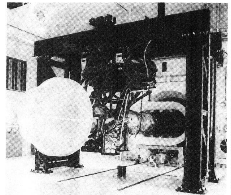
MOTEURS — Les engins qui équipent les chasseurs CF-18 sont testés sur un banc d'essai ultra-moderne. Lorsque le moteur F-404 qui développe 16,000 livres de poussée est sur le banc, l'ordinateur peut déceler la moindre faille dans ses entrailles.
