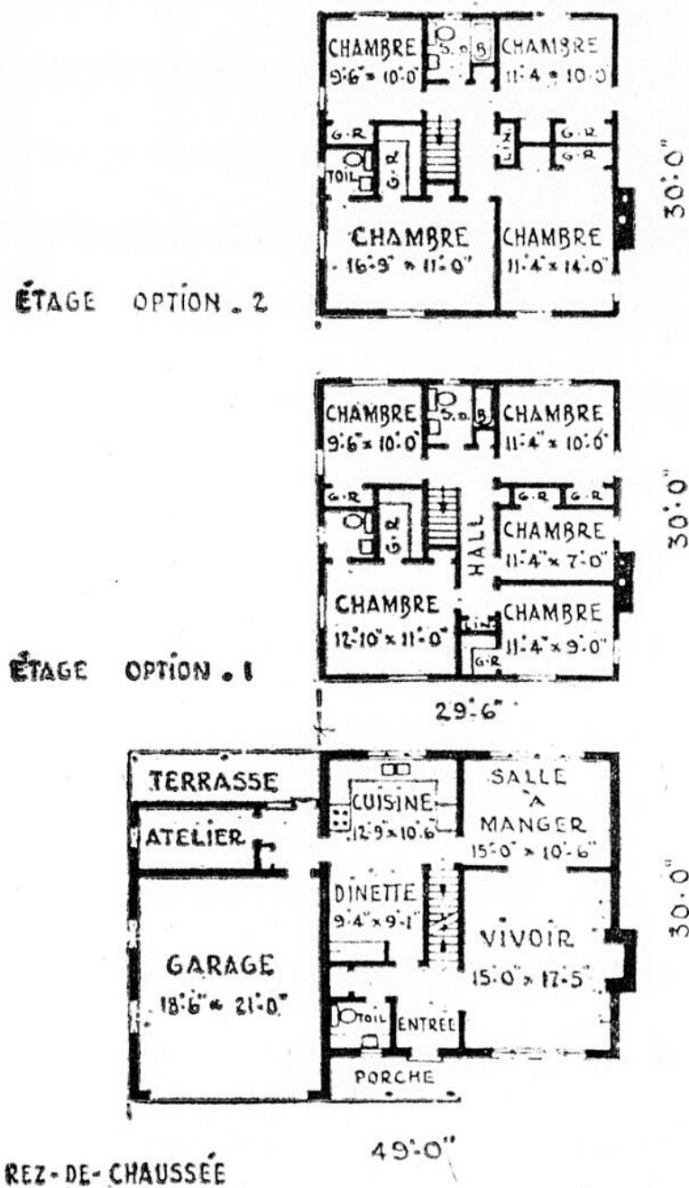
Plan du modèle P-CH-1078-F-B
