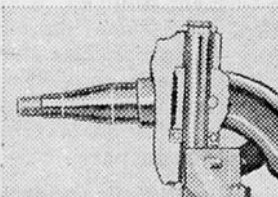
COUSSINETS DE NYLON SUR LES PIVOTS DE FUSÉES—Durent plus longtemps et ne nécessitent ni outils spéciaux ni manœuvres dans le cas d'un remplacement.
