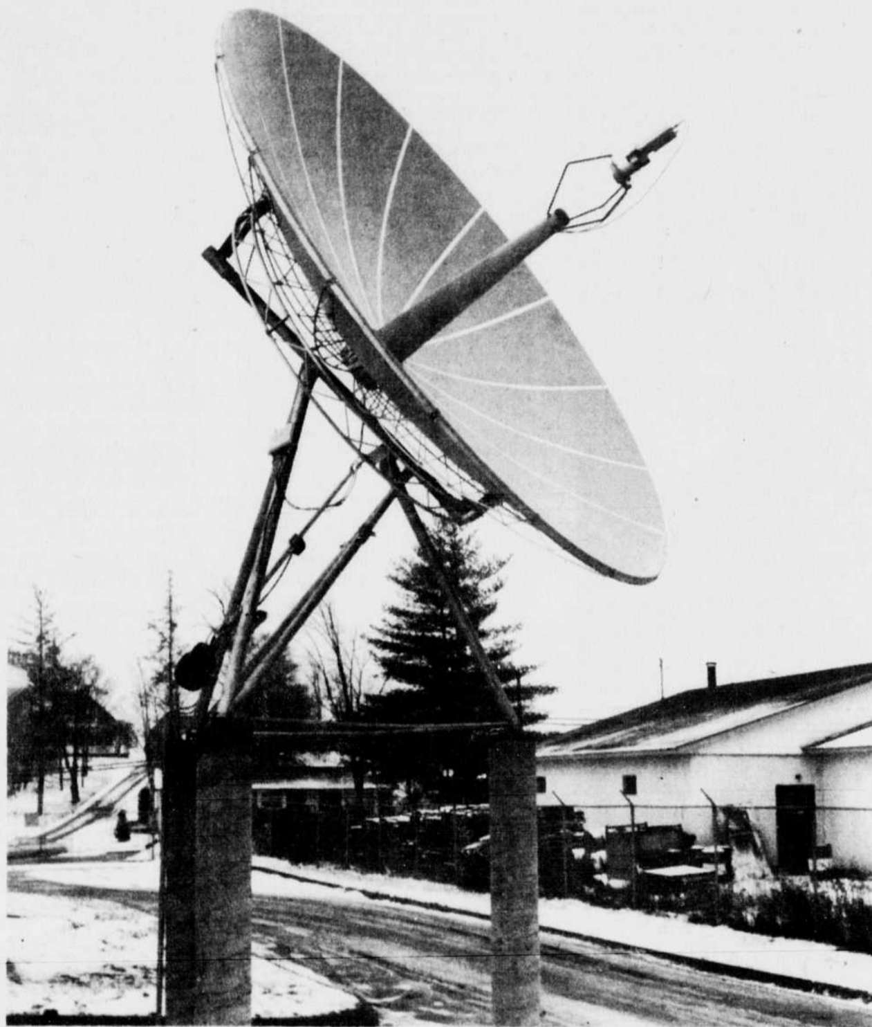
L'antenne parabolique de 3,6 m de diamètre seulement. L'ensemble ne pèse que 160 kilos. (Photo Gavroche)
