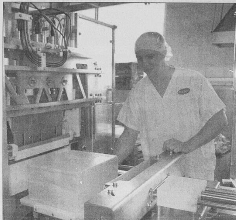
MACHINE - La Fromagerie Perron a investi 500 000 $ dans une nouvelle coupeuse. En moins de deux minutes, l'appareil tranche environ 50 pièces dans un bloc de 20 kilogrammes de fromage.
