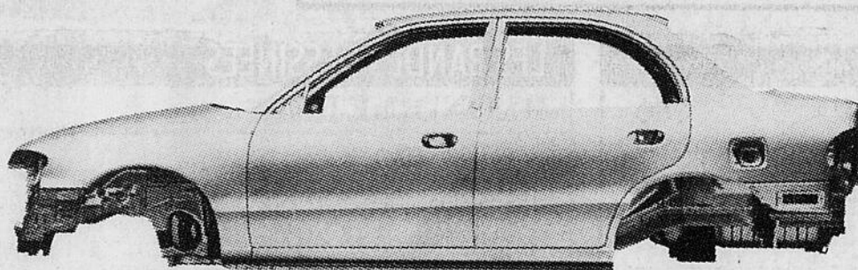
Des panneaux latéraux monopiece, en remplacement de panneaux en 6 pièces différentes, donnant à l'Accent plus d'homogénéité et de rigidité.
