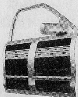
Deux poutrelles latérales de renfort pour une meilleure protection en cas d'impact latéral.
