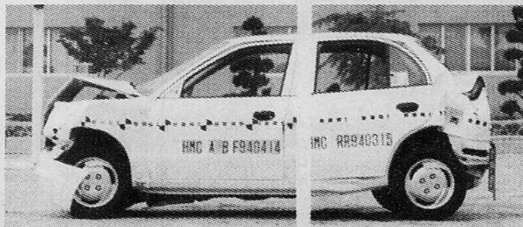
Zones déformantes avant et arrière conçues pour absorber le choc lors de collisions.
