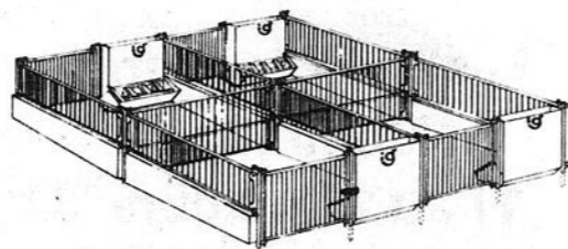
ENCLOS D'ENGRAISSEMENT EN TUYAU 1 5/8" D.E. HAUTEUR 36" TIGES 1/2" A 3 1/2" C/C OFFERTS GALVANISES OU PEINTURES
