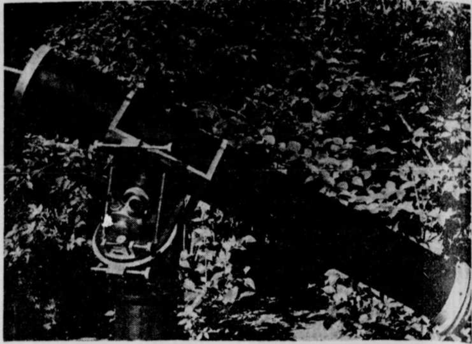
● Photographie du télescope de 6 pouces réalisé par M. L. McWilliams. La monture équatoriale Springfield a ceci de particulier que l'oculaire peut être toujours maintenu à une place fixe, c'est-à-dire sur une ligne parallèle à l'axe polaire. L'observateur se place dos au nord et face au sud et n'a à bouger que lorsqu'il utilise le chercheur.
