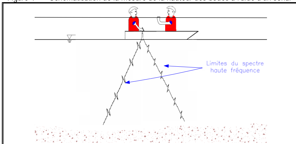
Figure 4 Schématisation de la mesure de la hauteur des boues à l'aide d'un sonar
