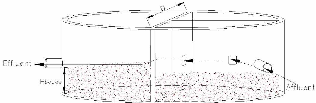
Figure 12 Exemple de bassin circulaire
