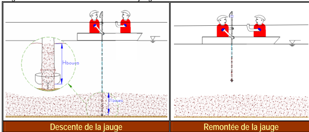
Figure 6 Descente et remontée de la jauge lors d'une mesure directe
