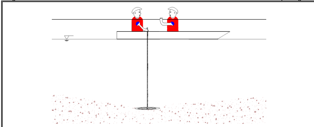
Figure 3 Schématisation de la mesure indirecte de la hauteur des boues avec un disque léger
