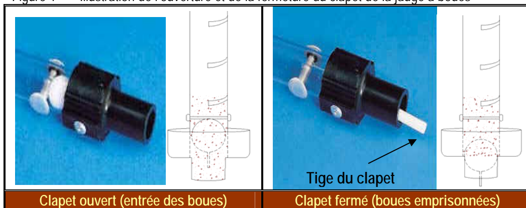
Figure 1 Illustration de l'ouverture et de la fermeture du clapet de la jauge à boues
