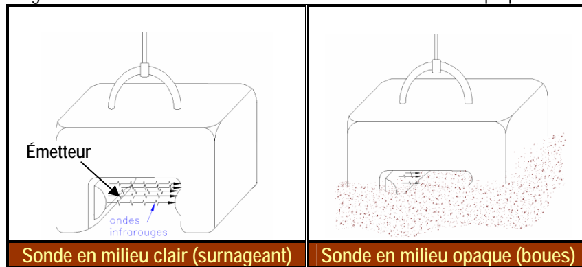
Figure 2 Illustration de la sonde en milieu clair et en milieu opaque
