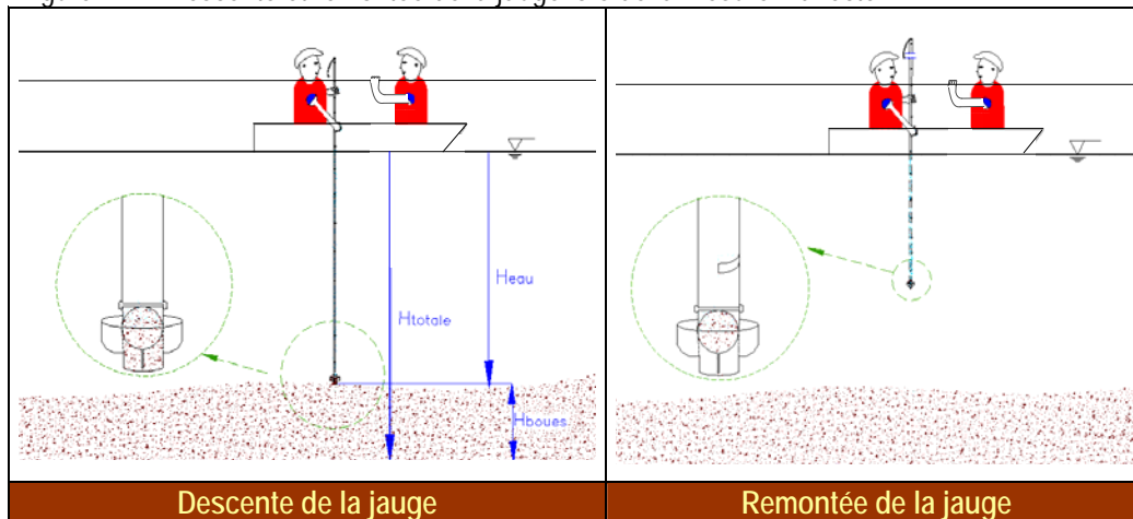
Figure 7 Descente et remontée de la jauge lors de la mesure indirecte
