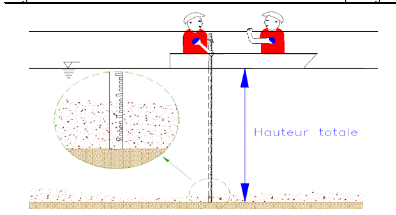
Figure 8 Mesure de la hauteur totale à l'aide d'une mire d'arpentage
