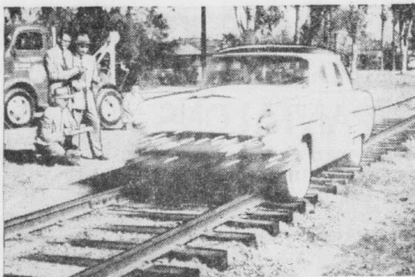
Ces pneus Super-Cushion, à cordes tout nylon, ont résisté à plus de 750.000 coups violents, au cours de longues journées de conduite sur des dormants de chemin de fer. Résultat étonnant: carcasses indemnes! Pas une corde rompue.
