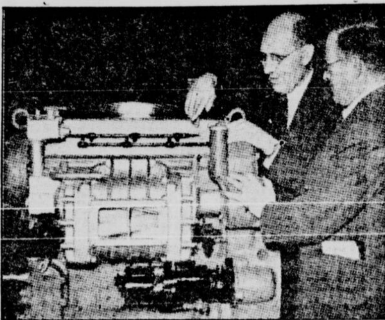
MM. KETTERING, à gauche, et R-K. EVANS, sont à examiner un moteur Diesel très léger, produit dans les usines de General Motors. Il n'est pas impossible qu'on voie ici le "moteur de demain".
