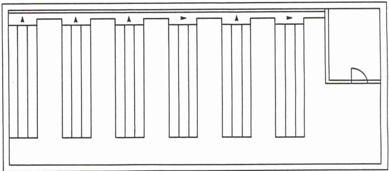
FIGURE 1 NETTOYEUR À CLAPIER, ARRANGEMENT GÉNÉRAL
