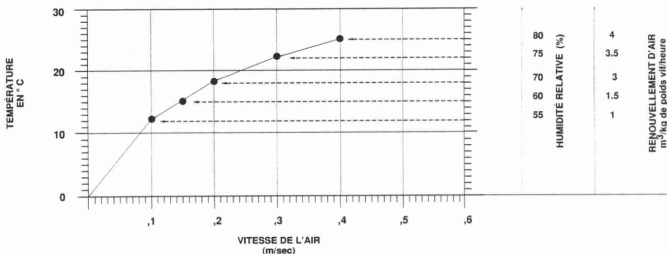
Graphique 1: Relations entre la température, la vitesse de l'air, l'humidité relative et le renouvellement d'air
