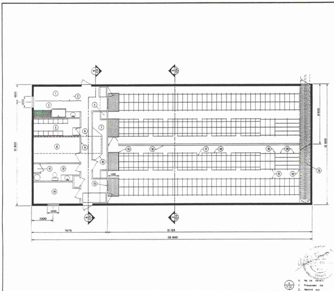
FIGURE 2 CLAPIER MIXTE (FLAT DECK), 100 CAGES MÈRES
