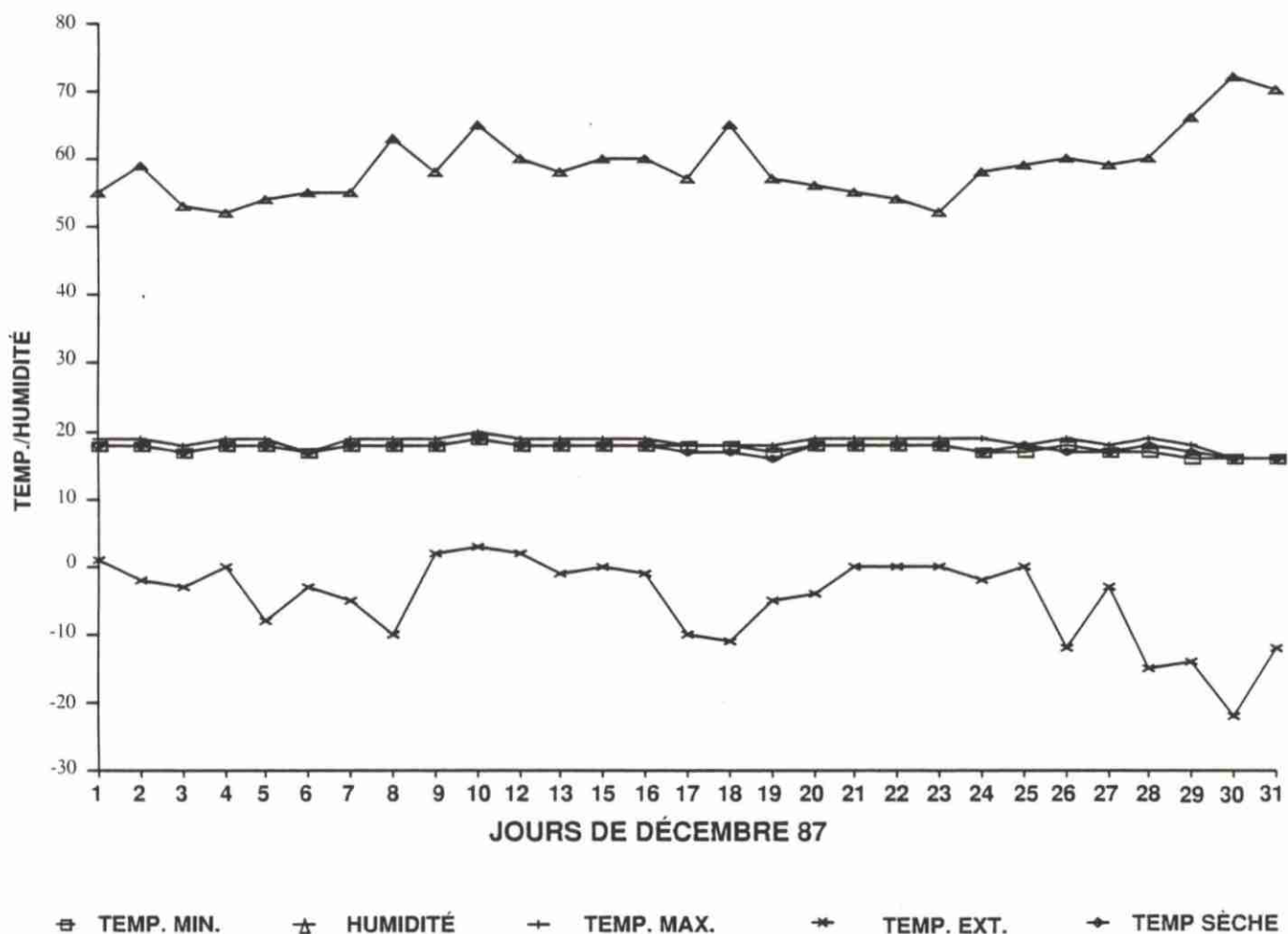
FIGURE 2 CLAPIER DESÈVE, SALLE MIXTE VARIATION DE LA TEMPÉRATURE ET DE L'HUMIDITÉ EN DÉCEMBRE.
