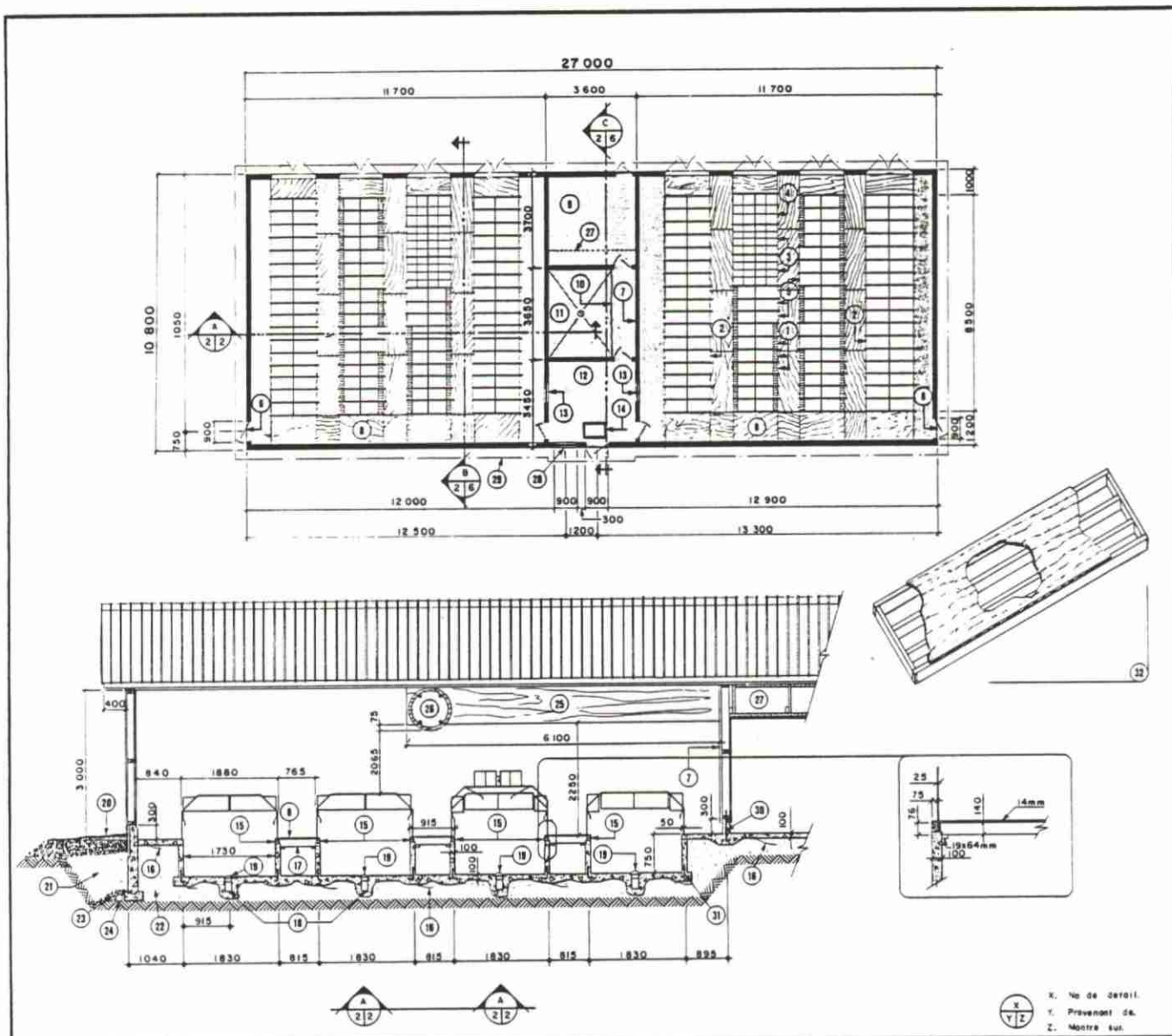
FIGURE 3 CLAPIER MIXTE À FOSSES SEMI-PROFONDES, 92 CAGES MÈRES
